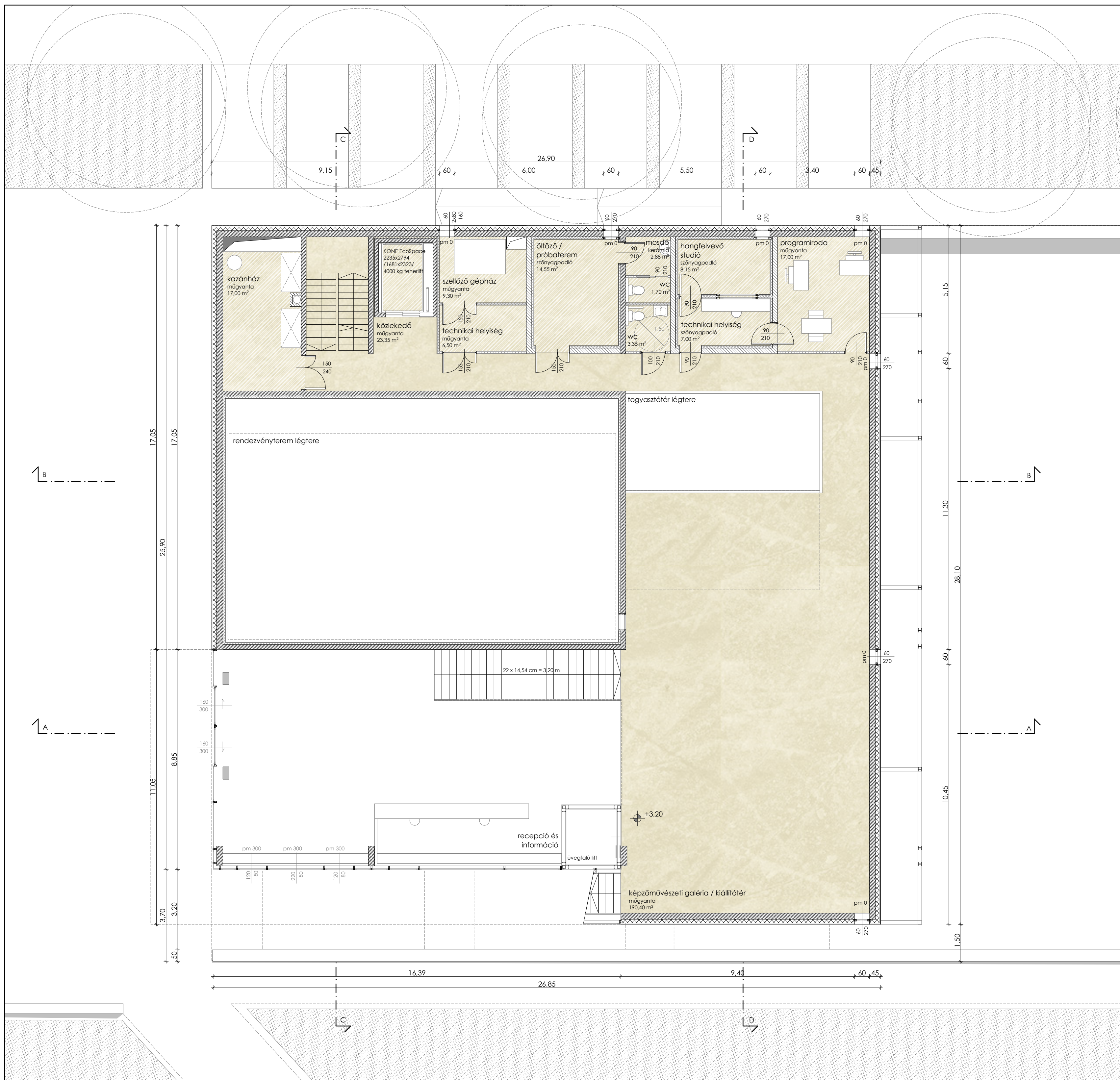
GALÉRIA ALAPRAJZ M=1:100
