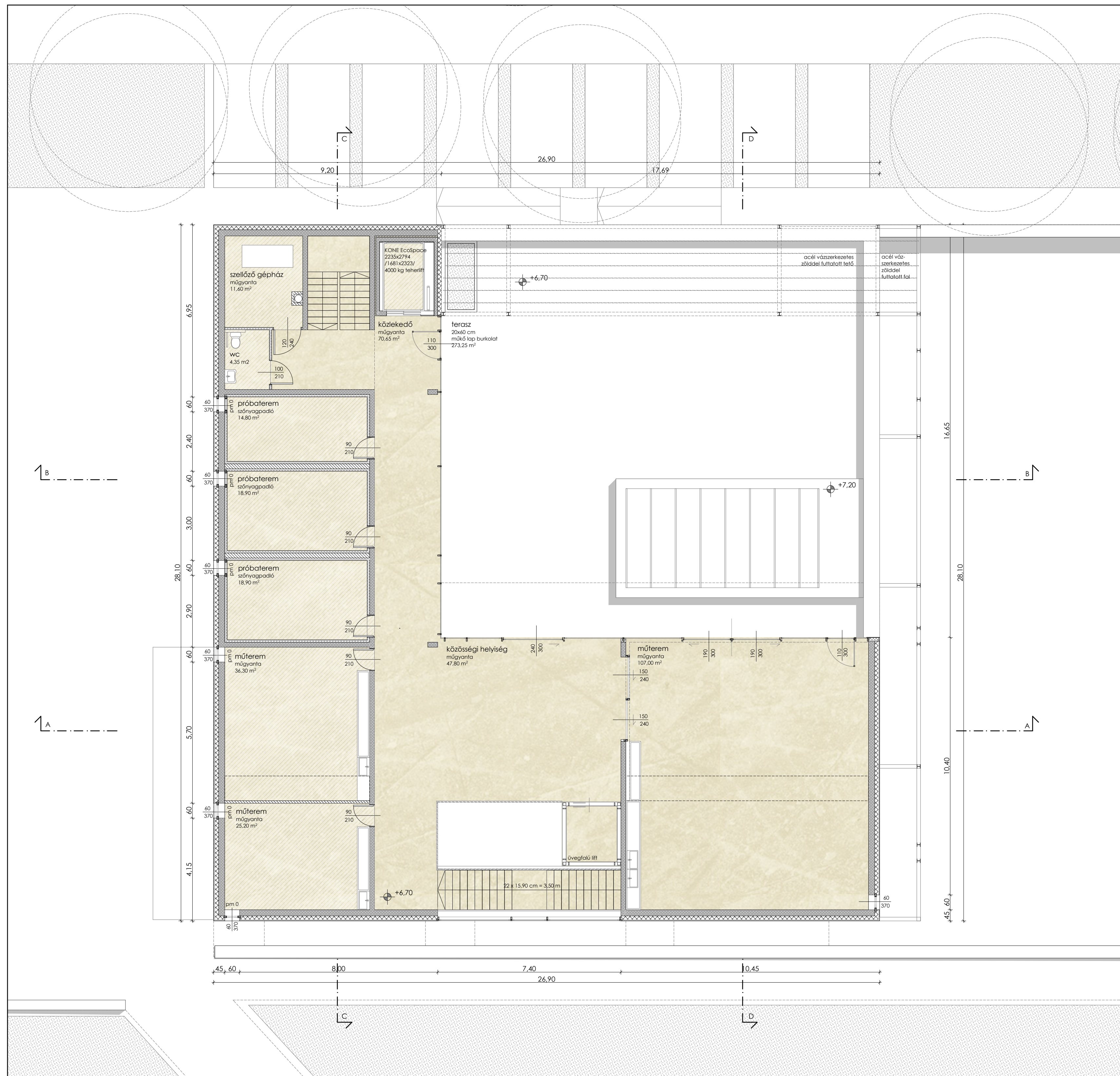
EMELETI ALAPRAJZ M=1:100
