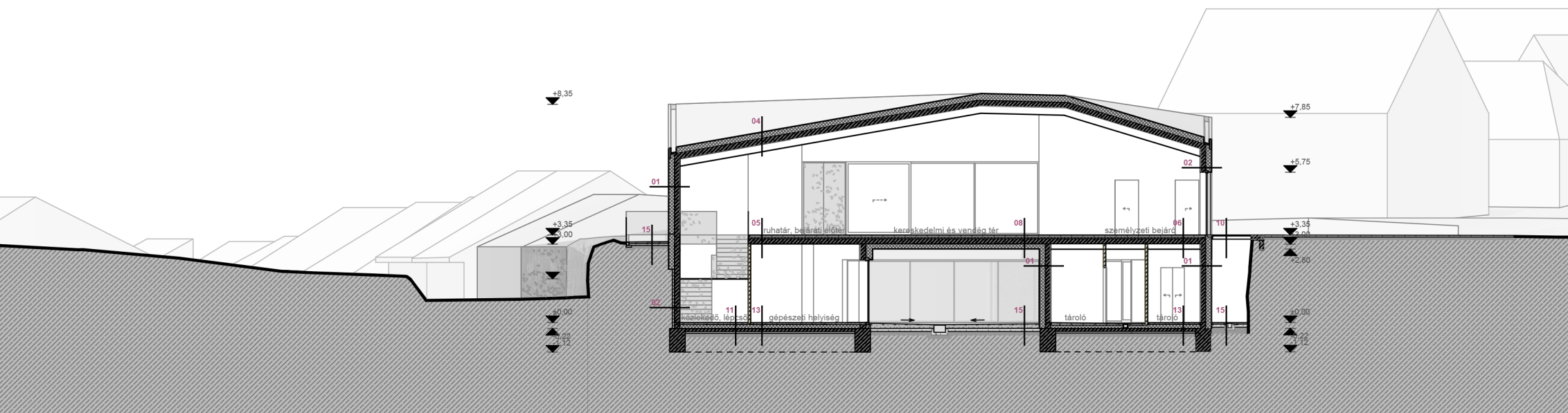
1 2 10 20m 05 . KURFIS ALÍZ EDIT . MAGOLAJHÁZ - MOGYORÓD . SZIE-YMMF MSC . . DIPLOMATERV 2013 ..... C-C, D-D METSZET. M 1:200 .
