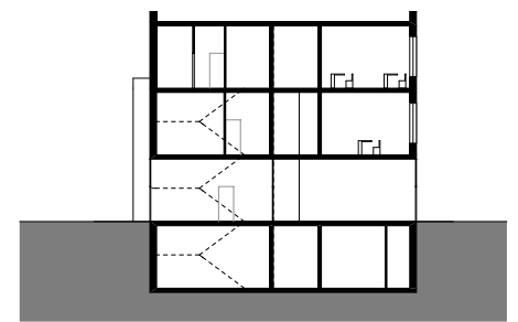
2-2 metszet
