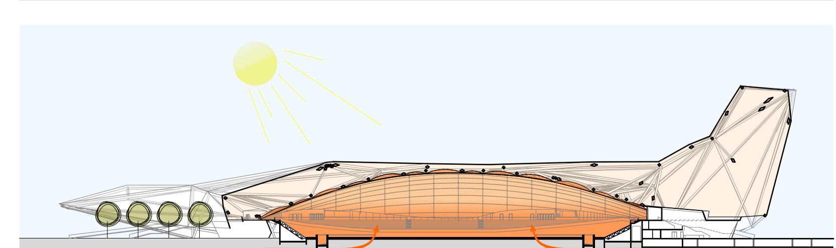
A velodrom nyári és téli fenntartható temperáló-szellőztető rendszere
