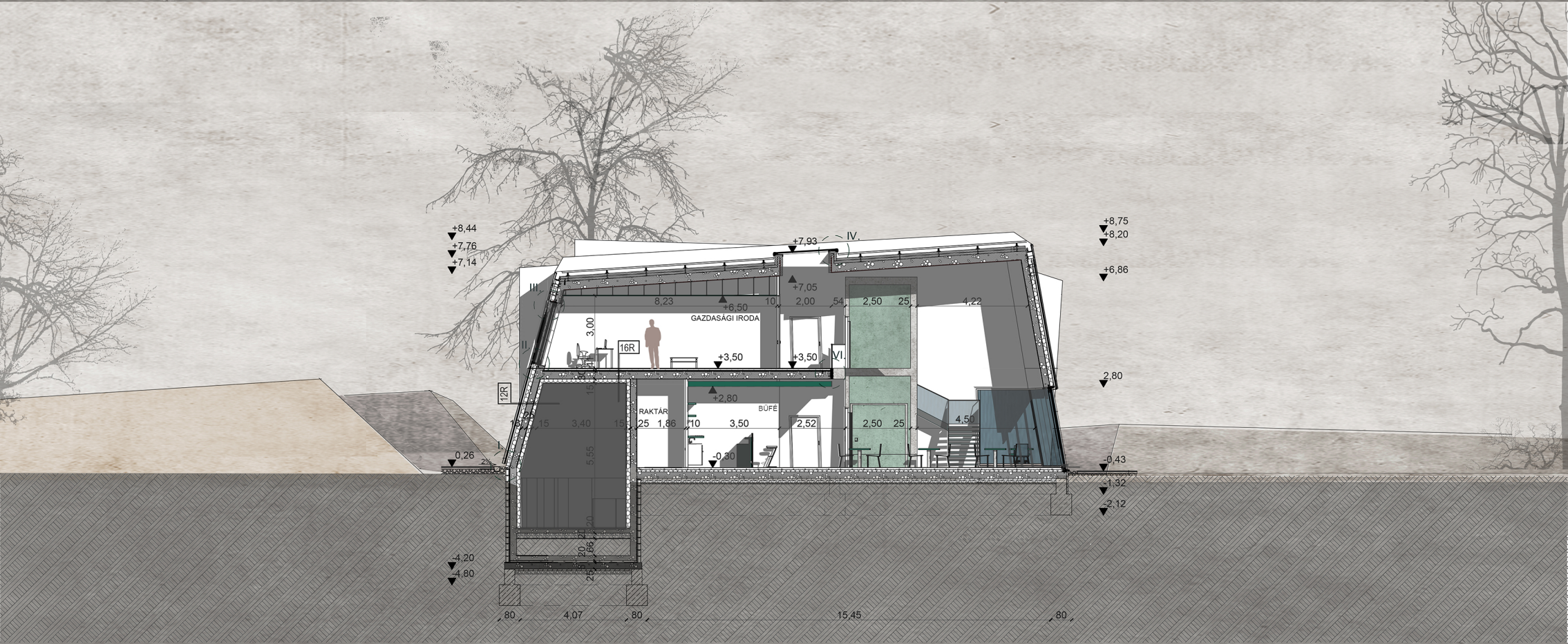
B-B METSZET M=1:100
