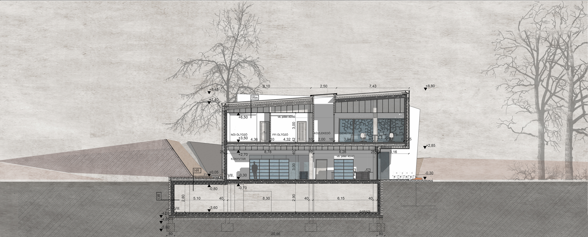
C-C METSZET M=1:100
