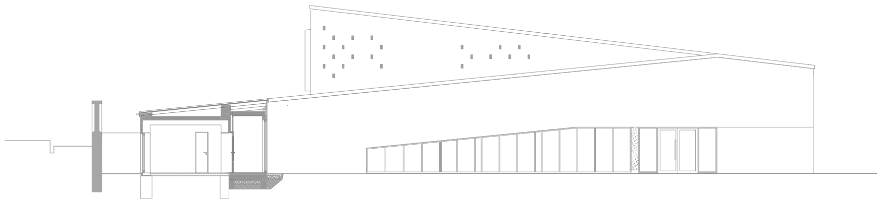
G-G METSZET
