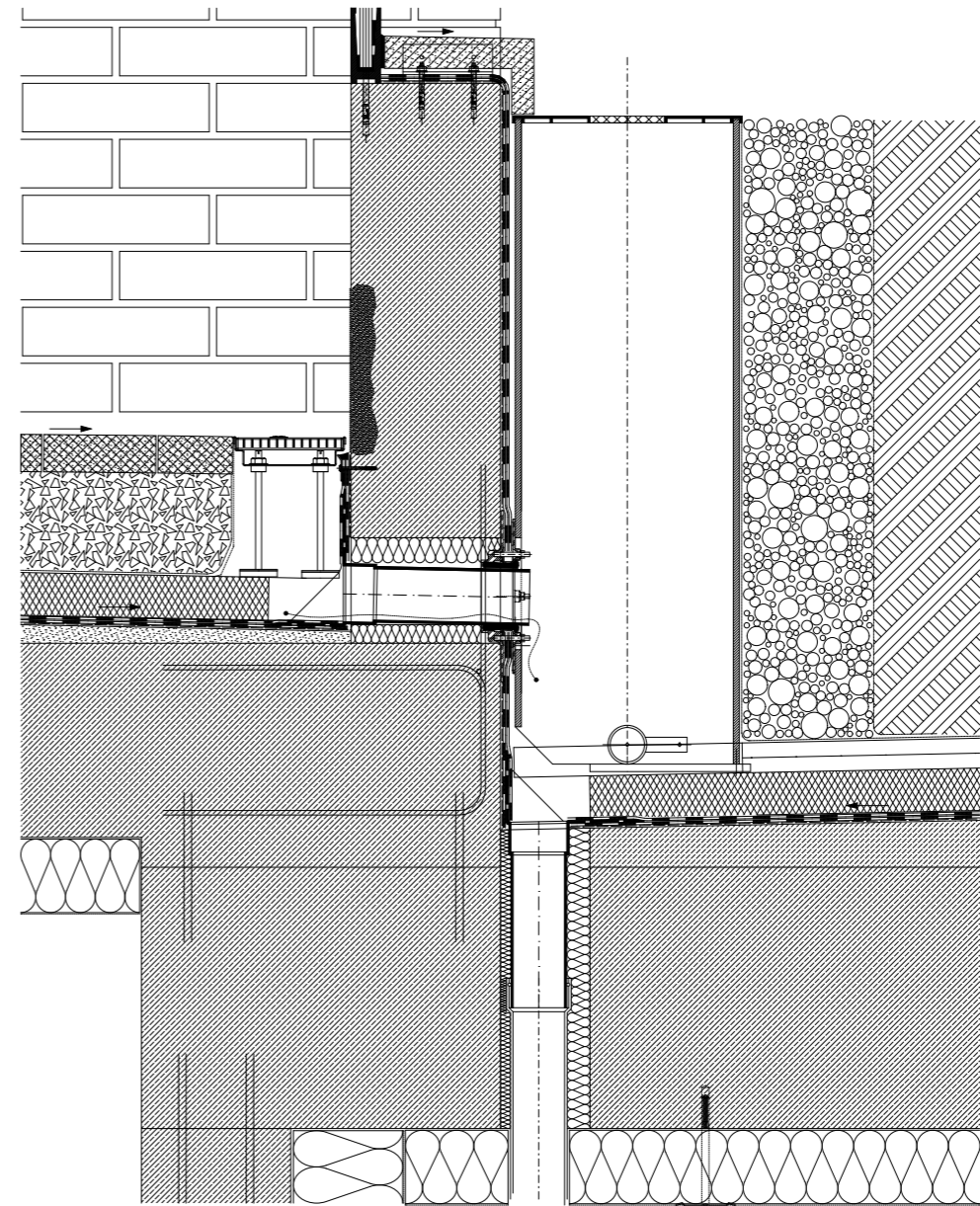
Somogyi Könyvtár felőli terasz és zöldtető összefolyójának kapcsolata a földszinten
