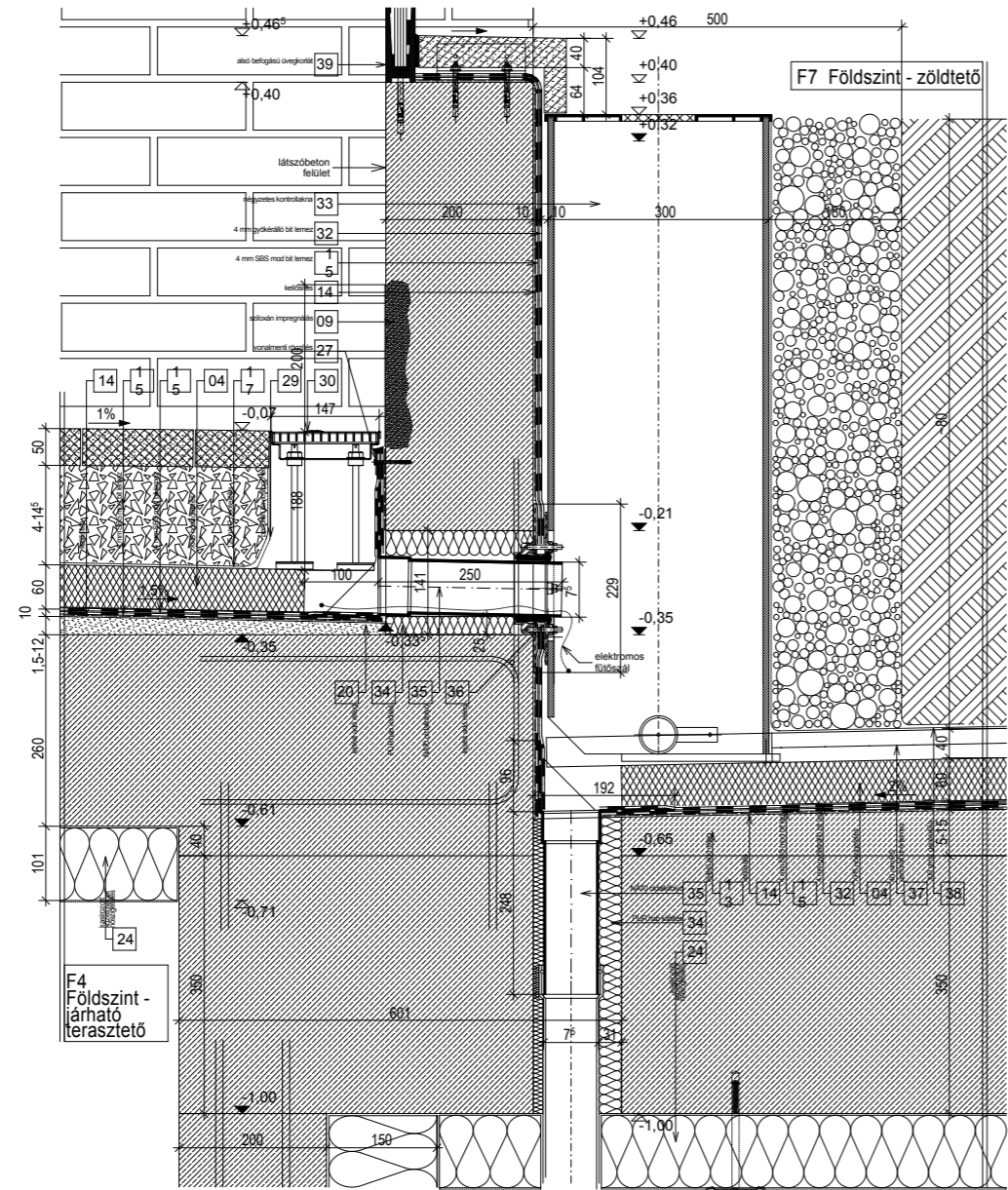
Somogyi Könyvtár felőli terasz és zöldtető összefolyójának kapcsolata a földszinten
