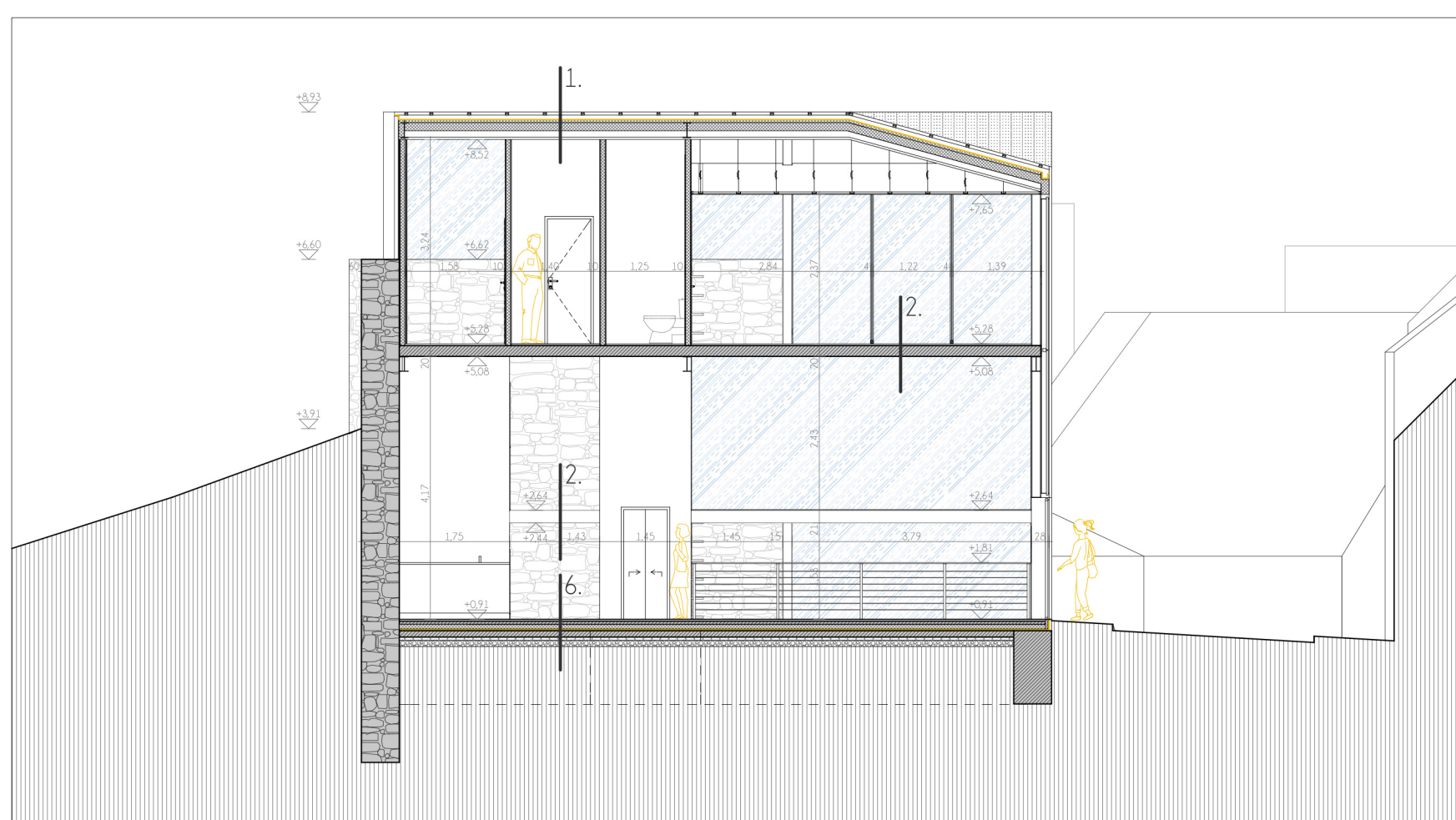
B - METSZET M 1:100
