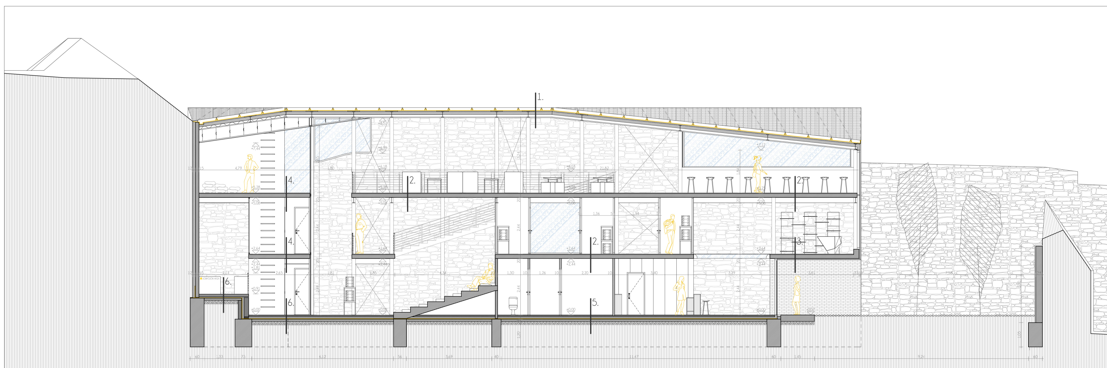
A - METSZET M 1:100
