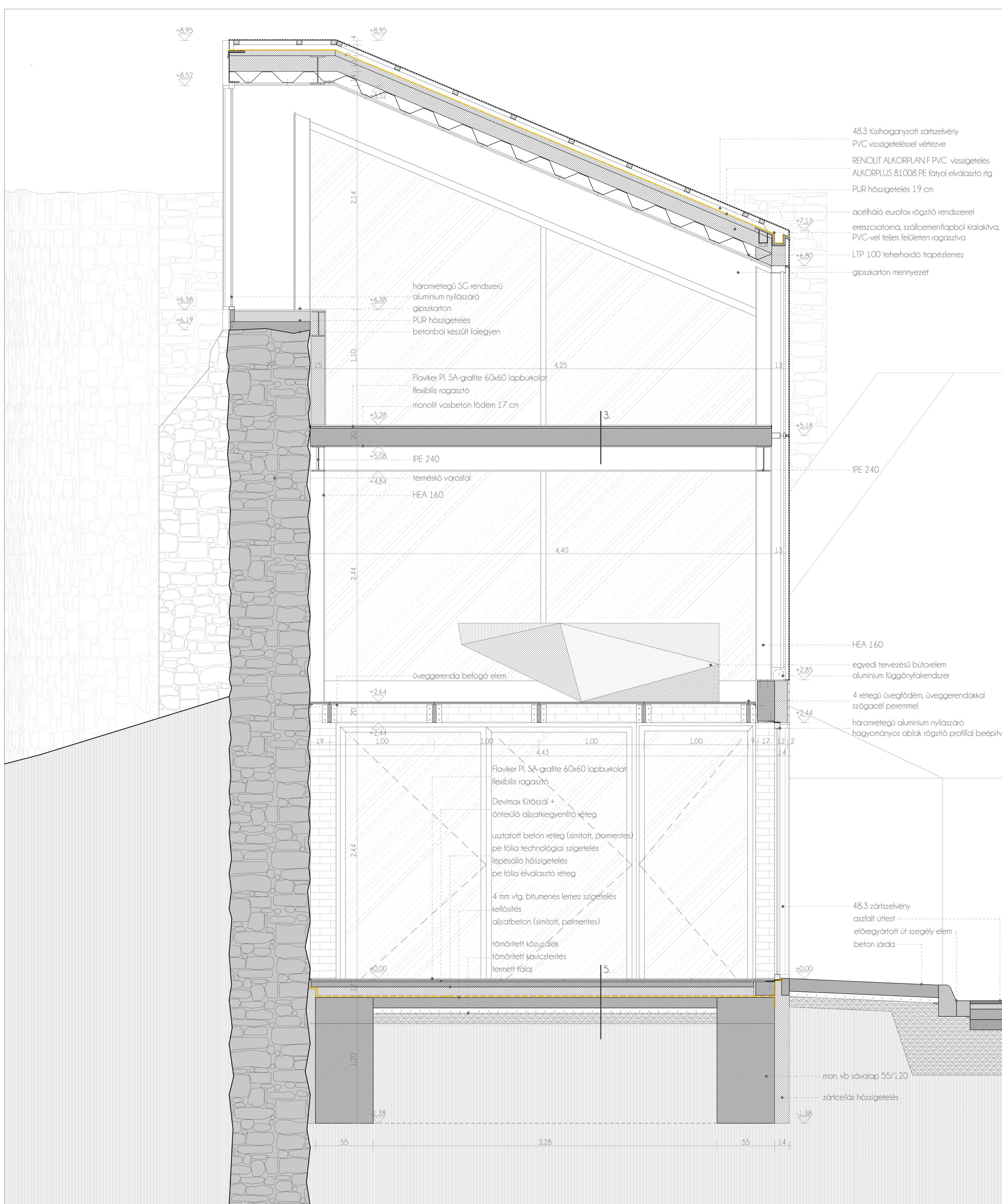
D - FŐFALMETSZET M 1:20
