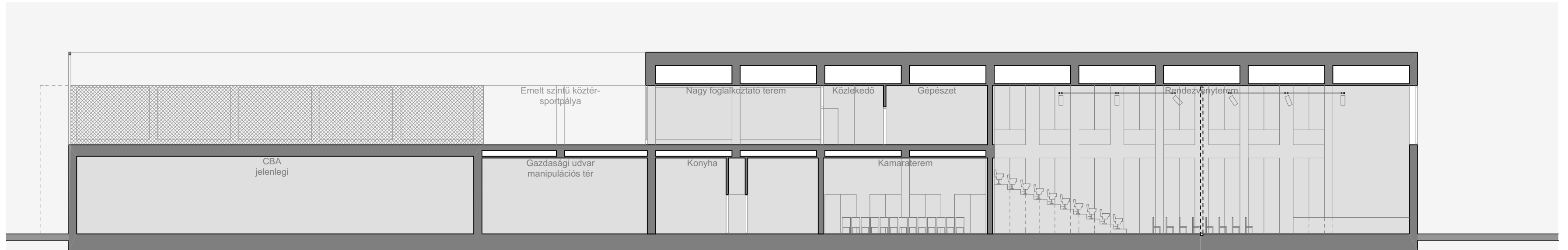
D-D METSZET M 1:200
