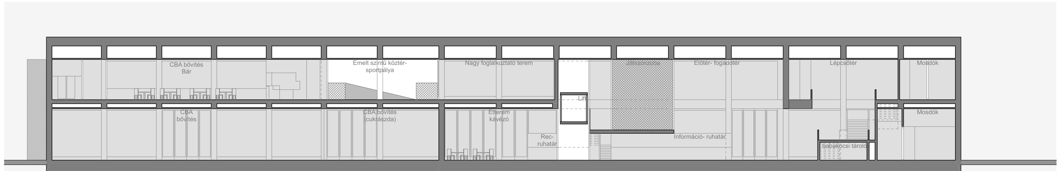
E-E METSZET M 1:200
