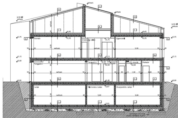
"C-C" metszet
