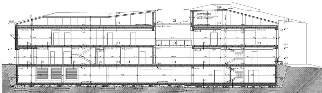
"A-A" metszet
