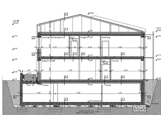
"B-B" metszet
