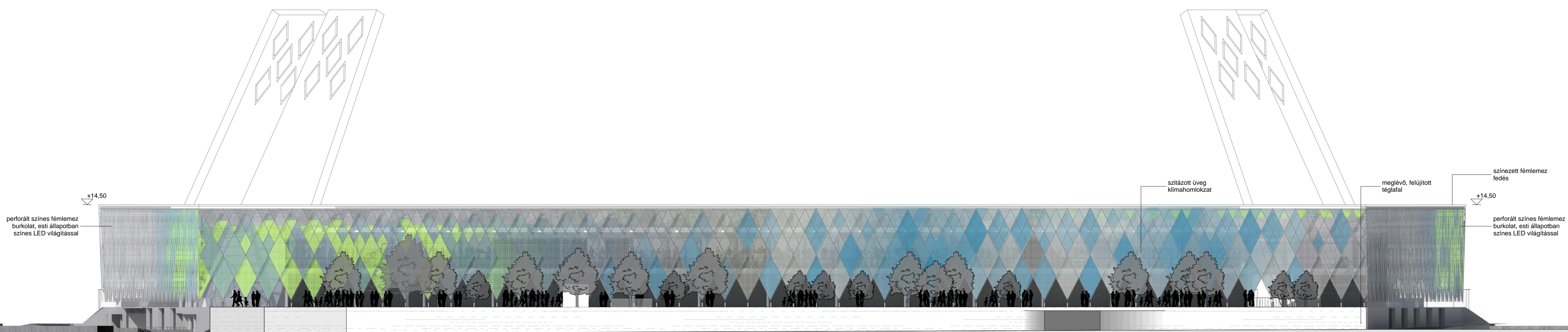
NYUGATI HOMLOKZAT M 1:250
