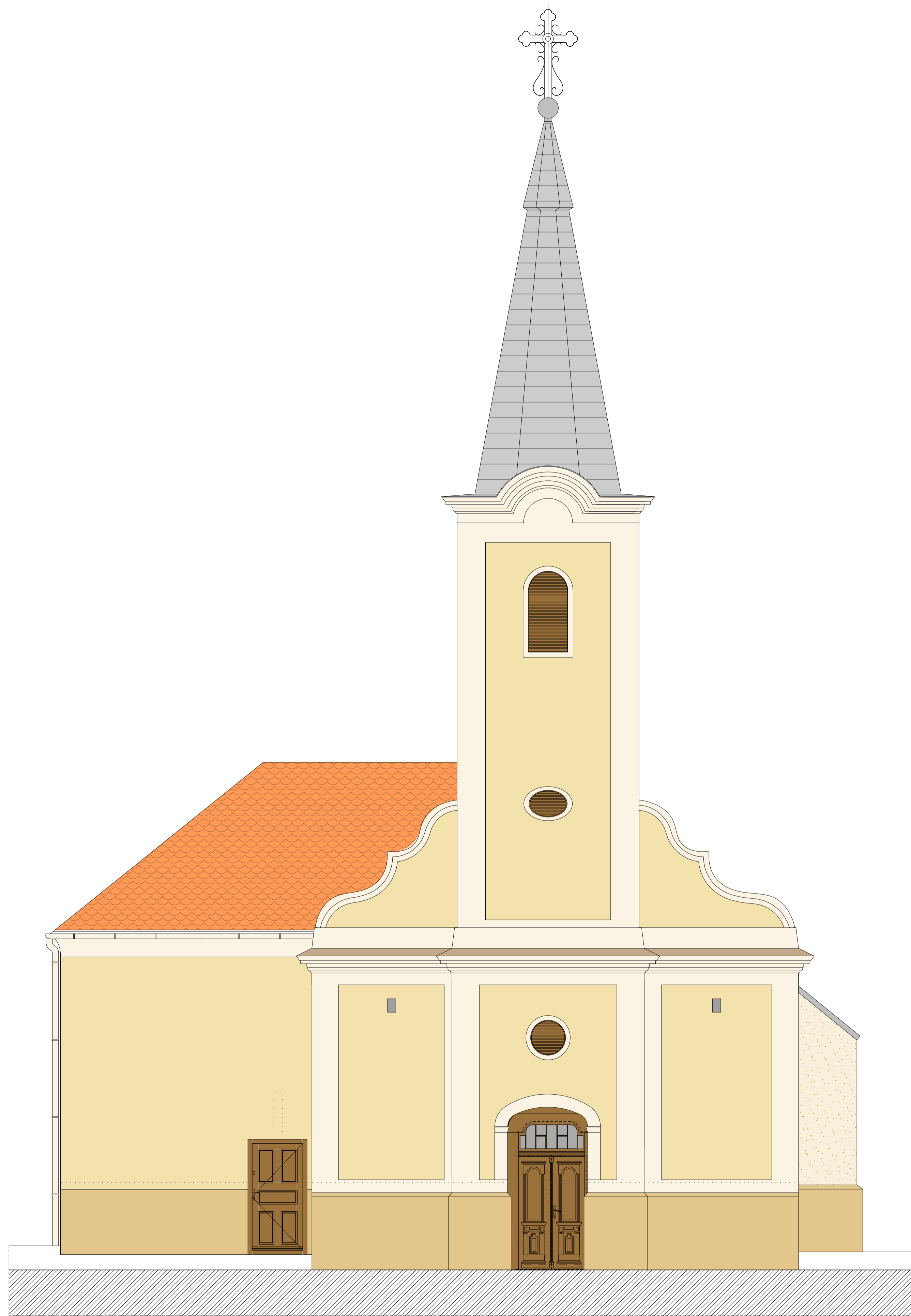
Tervezett nyugati homlokzat M 1:50
