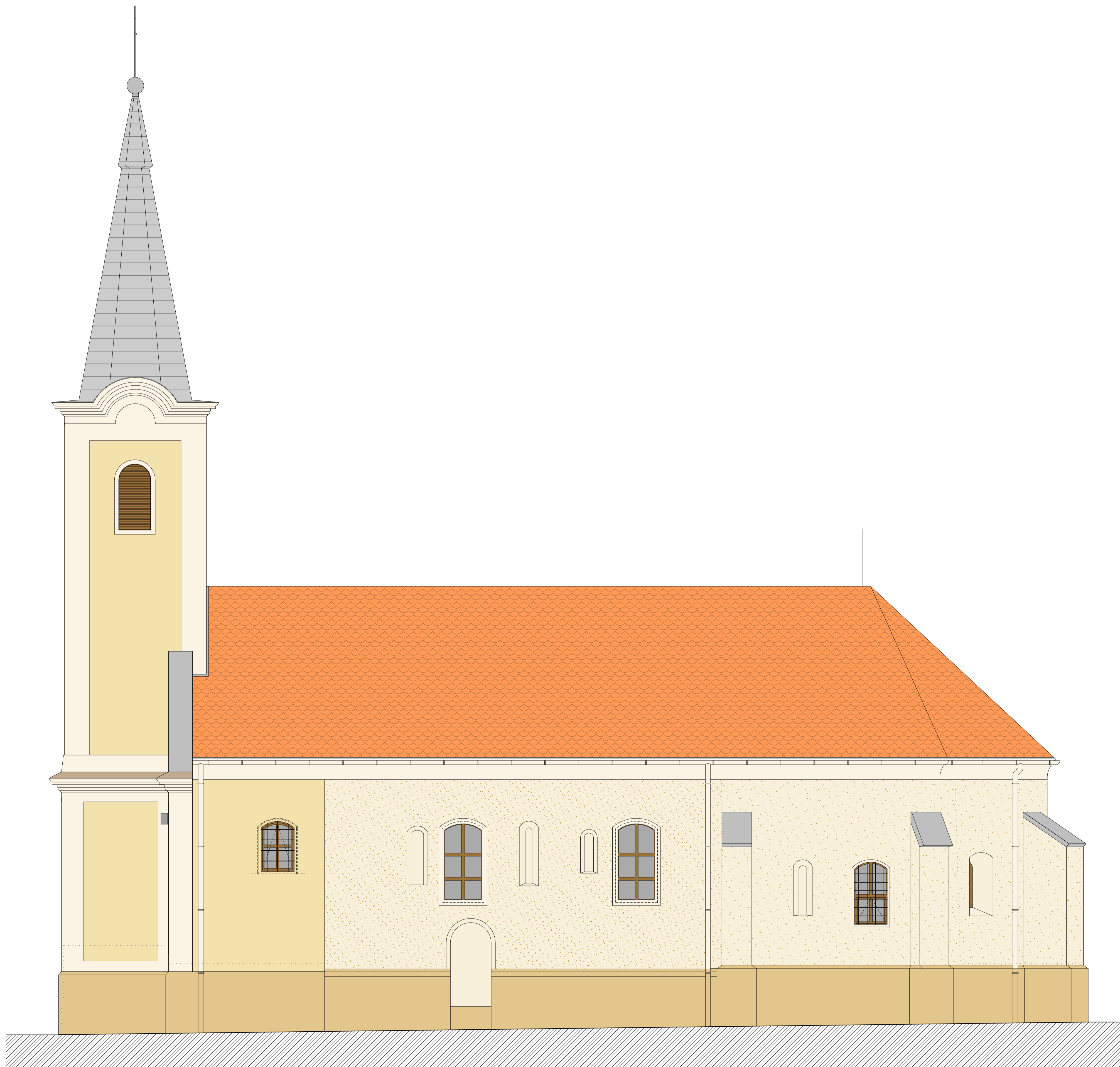
Tervezett déli homlokzat M 1:50
