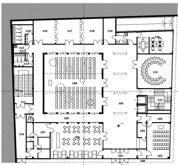
FÖLDSZINT ALAPRAJZA
