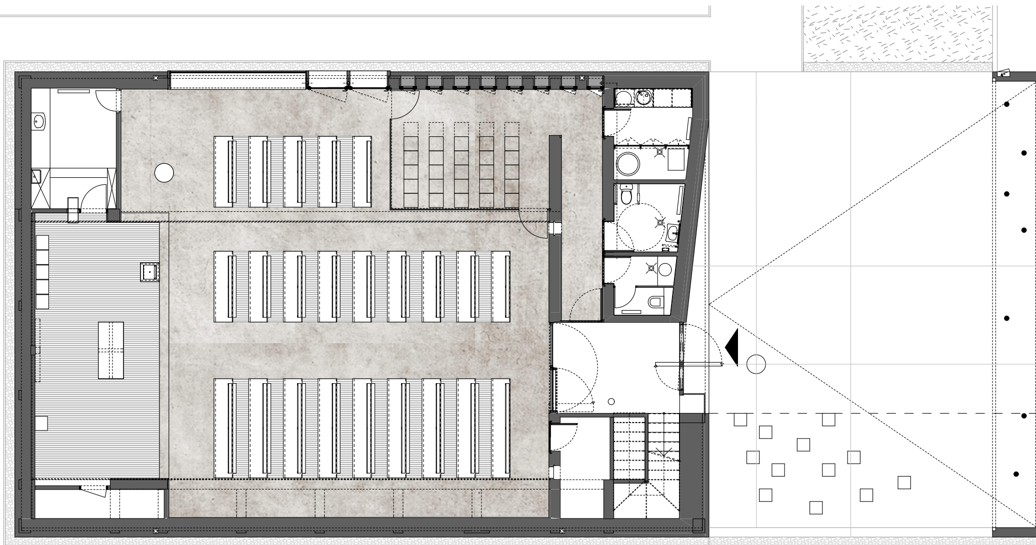
FÖLDSZINTI ALAPRAJZ
