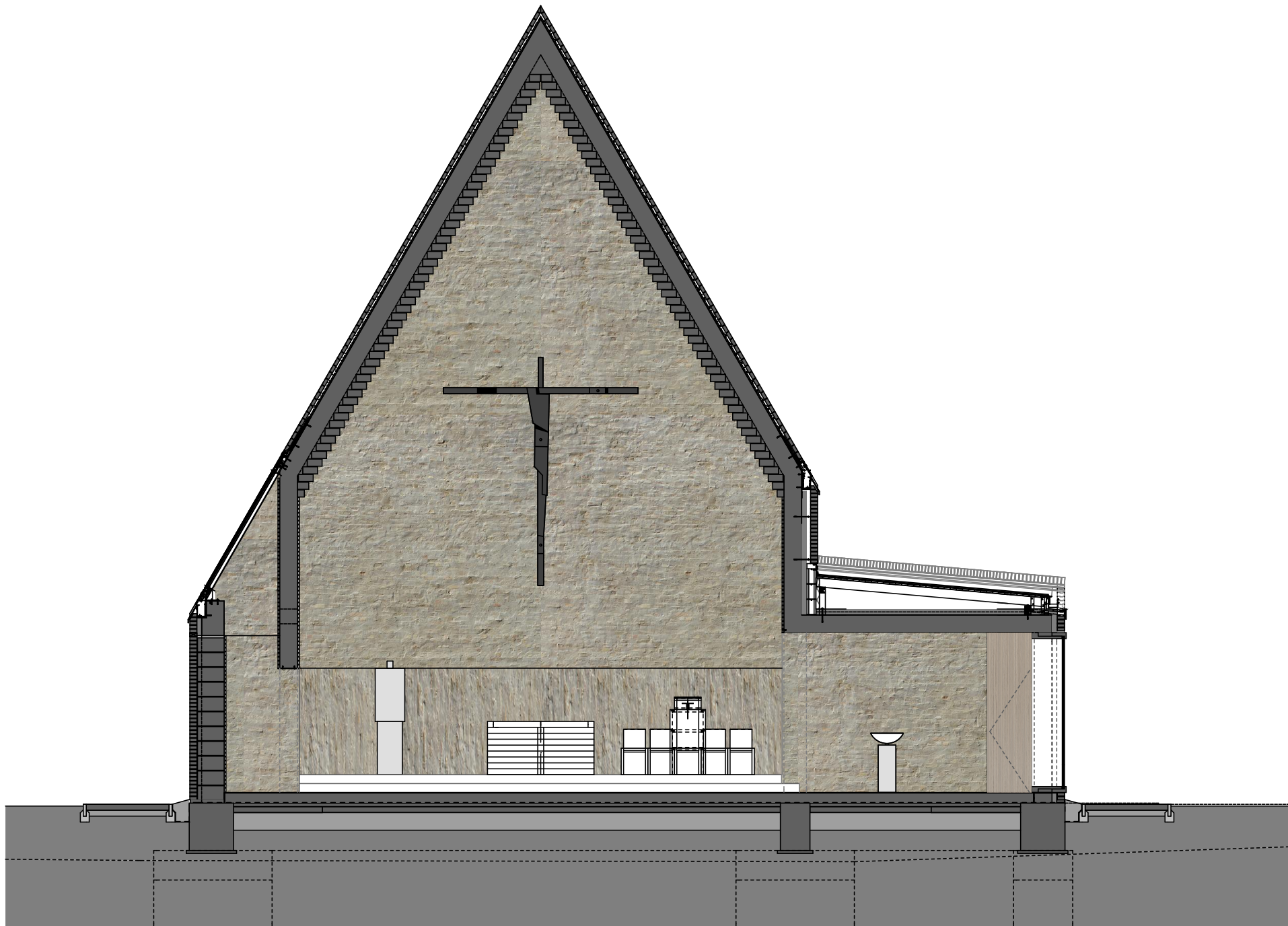
A-A METSZET
