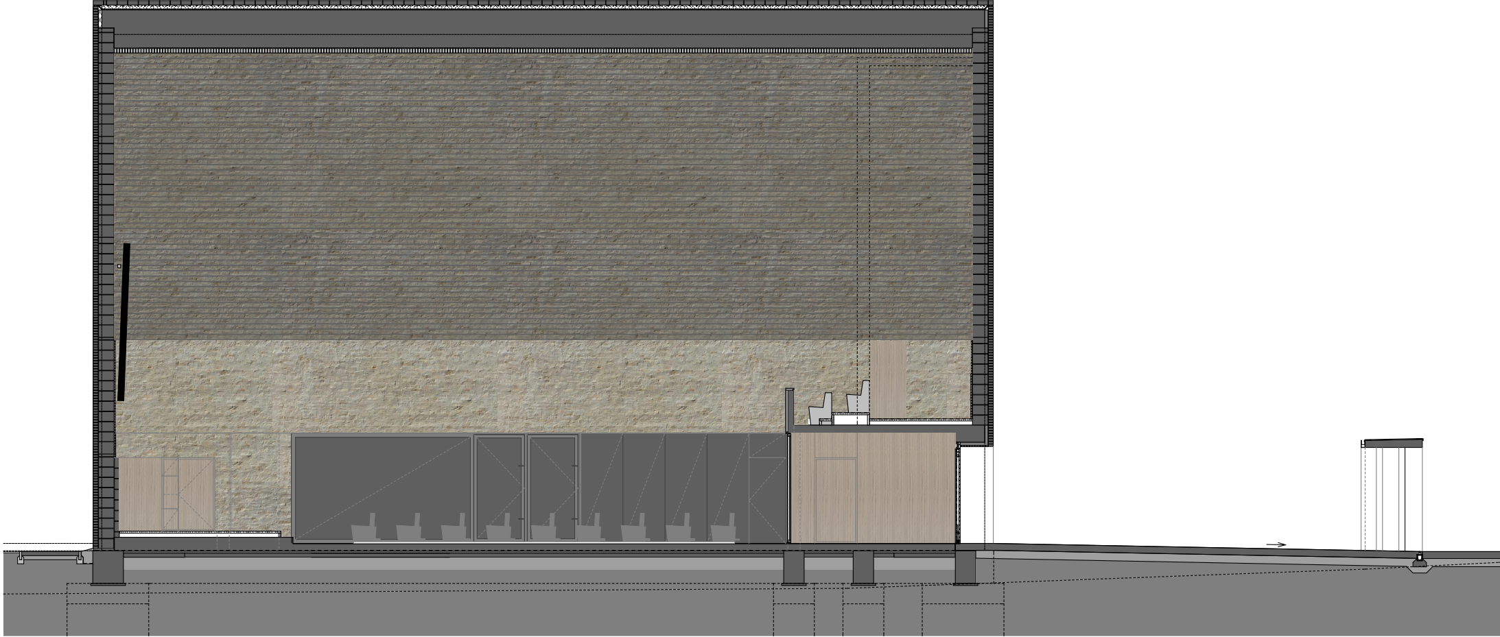
B-B METSZET
