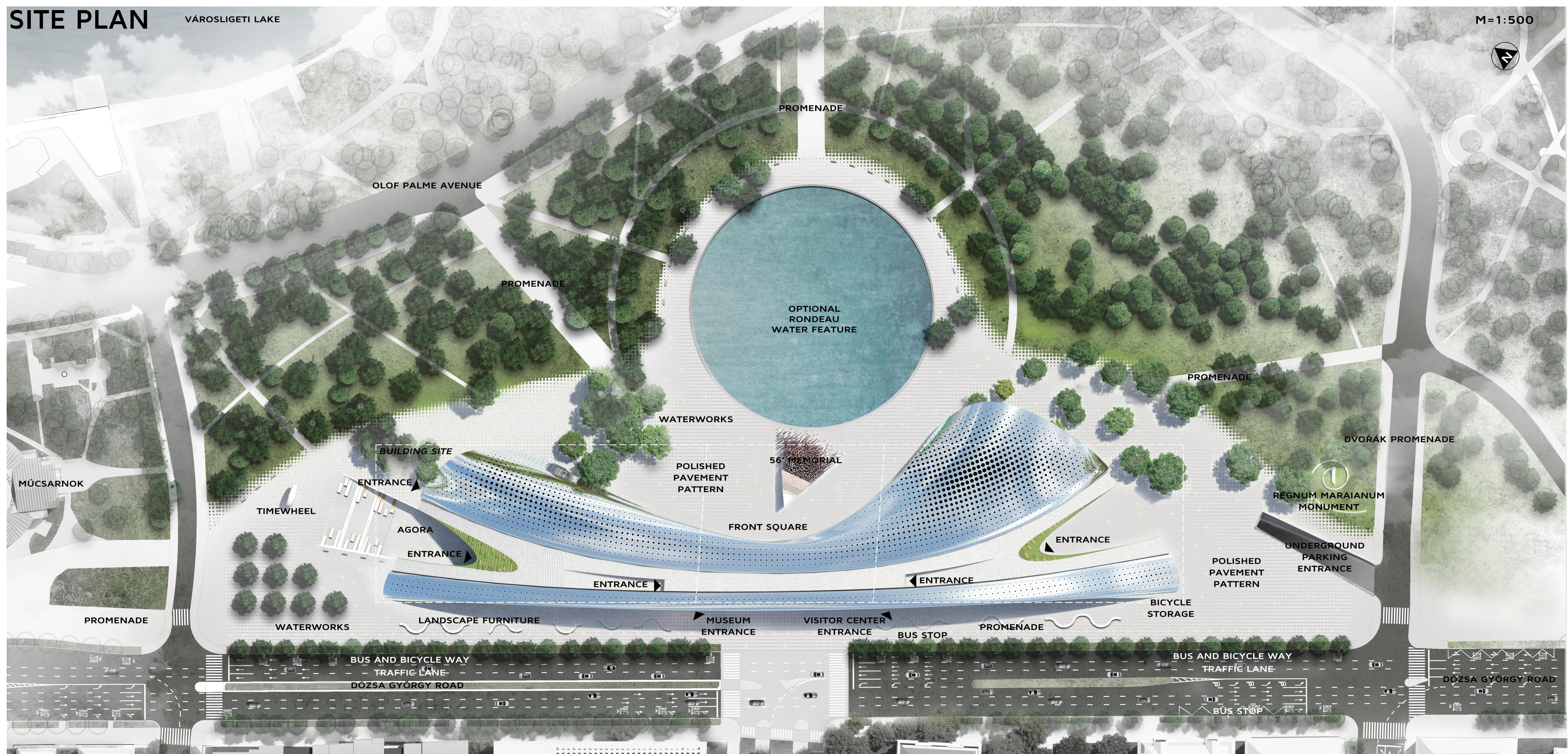
SITE PLAN 1/500
