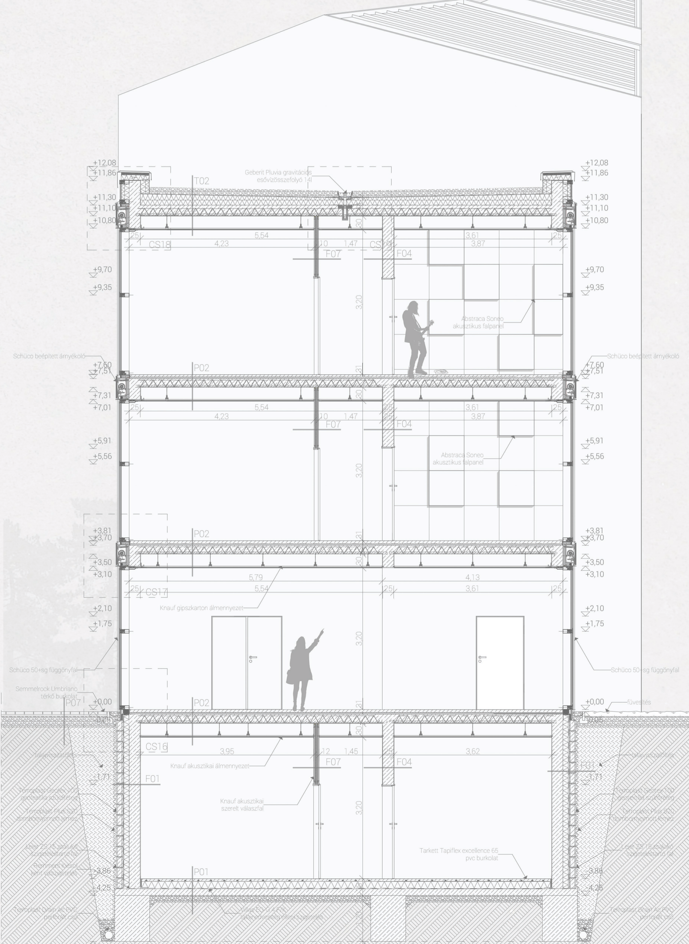
b-b metszet m1:50
