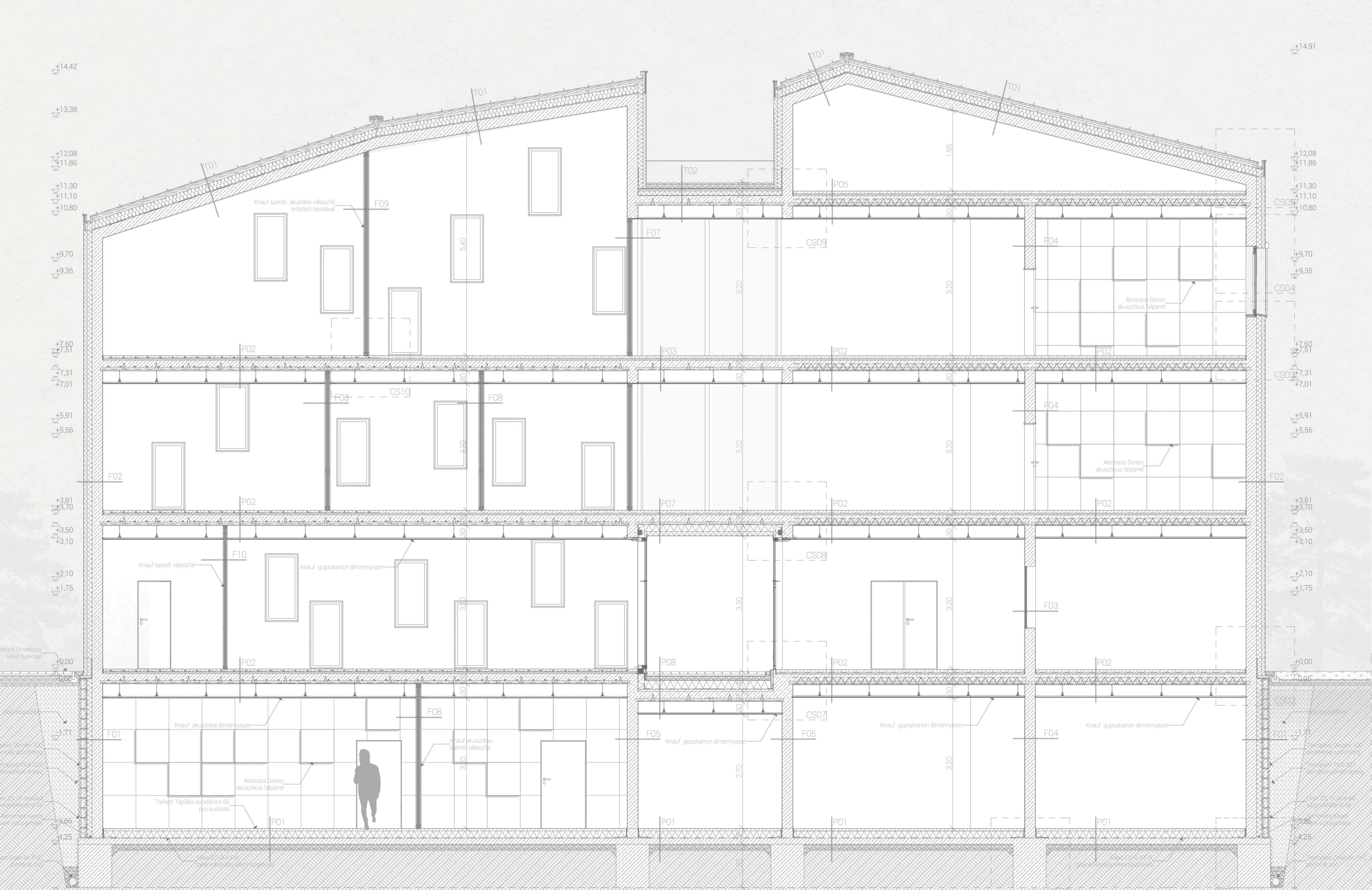
c-c metszet m1:50
