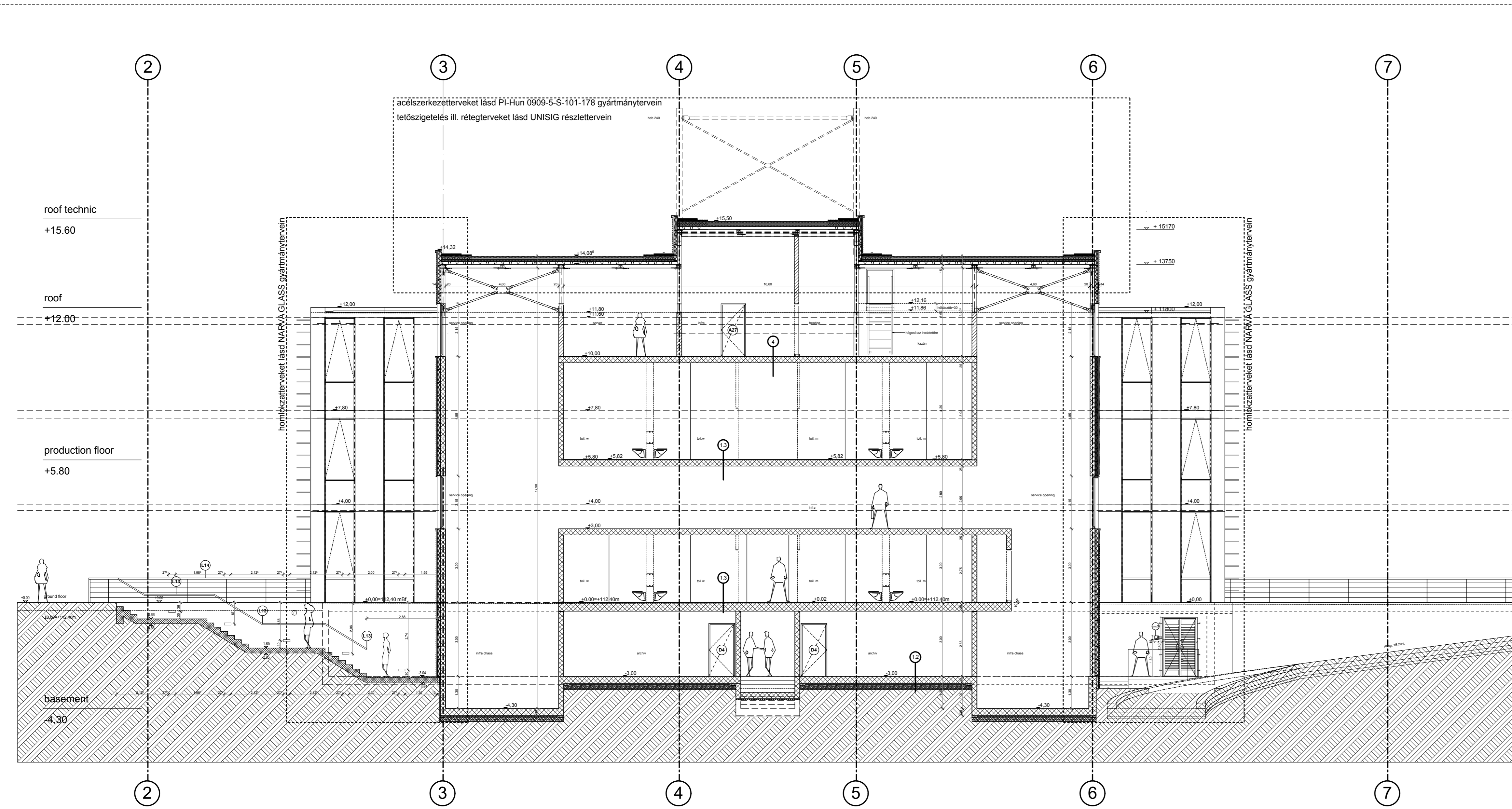
longitudinal section 4-4
