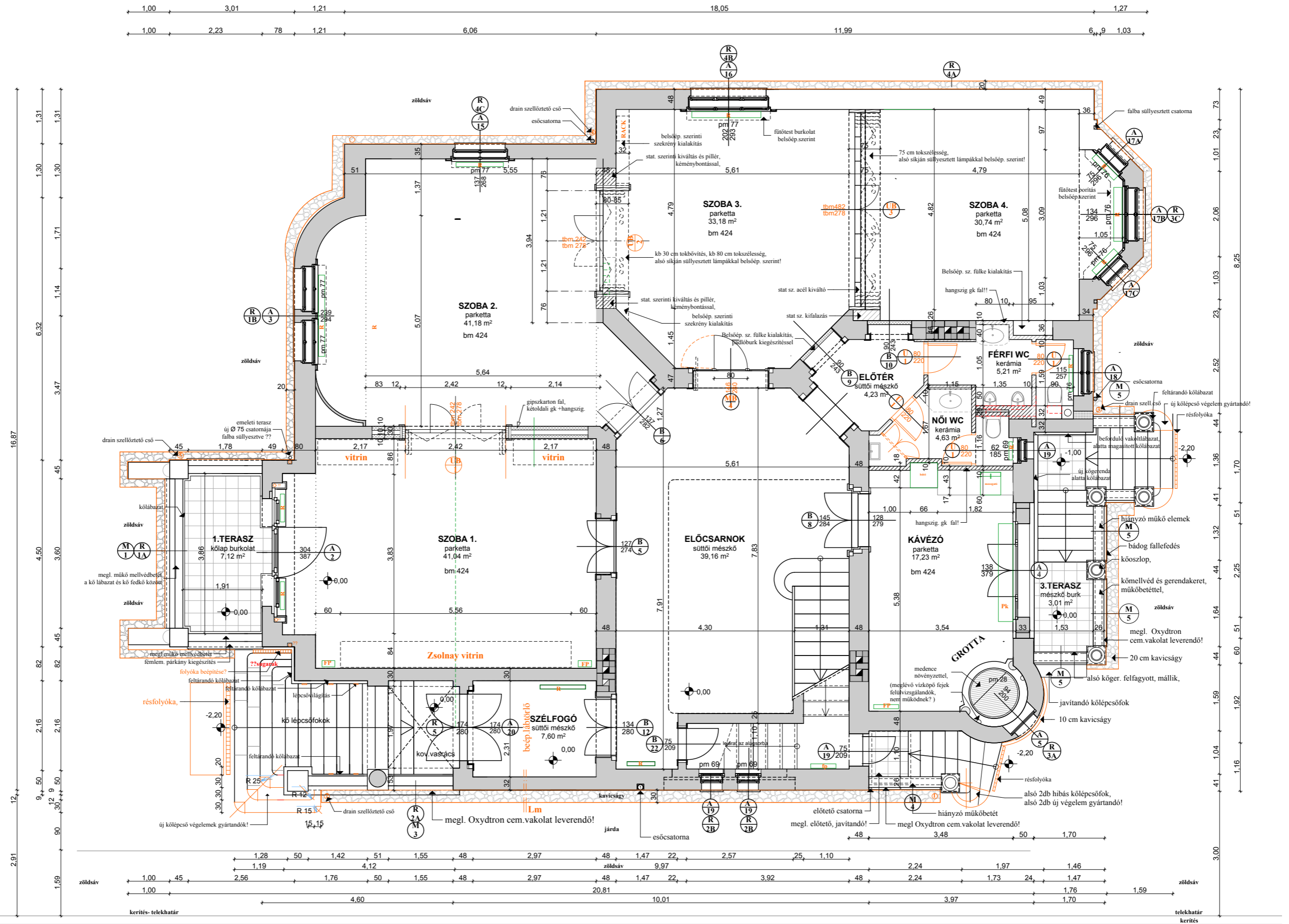
FÖLDSZINTI ALAPRAJZ (ÉPÍTÉS)
