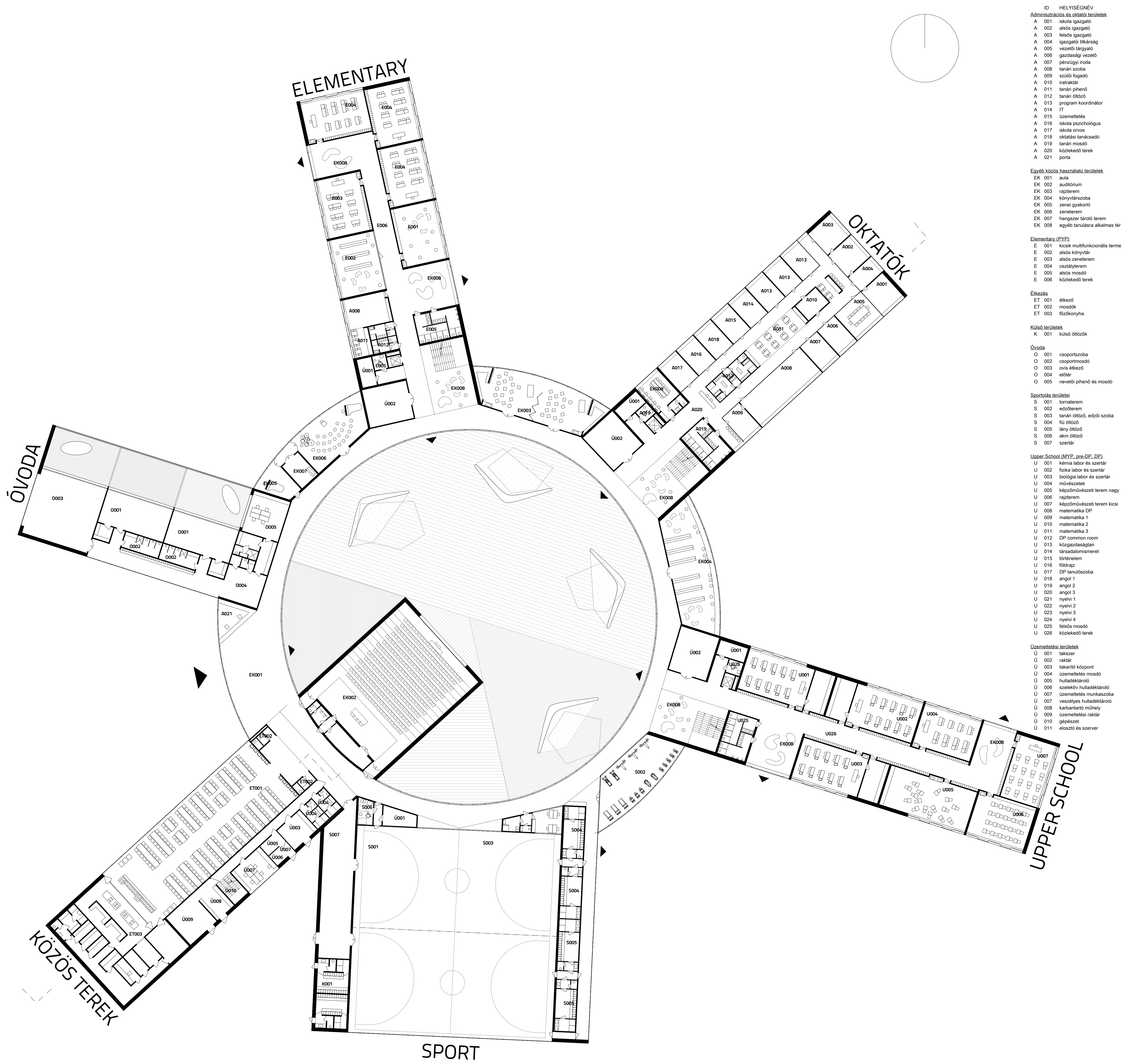
FÖLDSZINTI ALAPRAJZ 1_250
