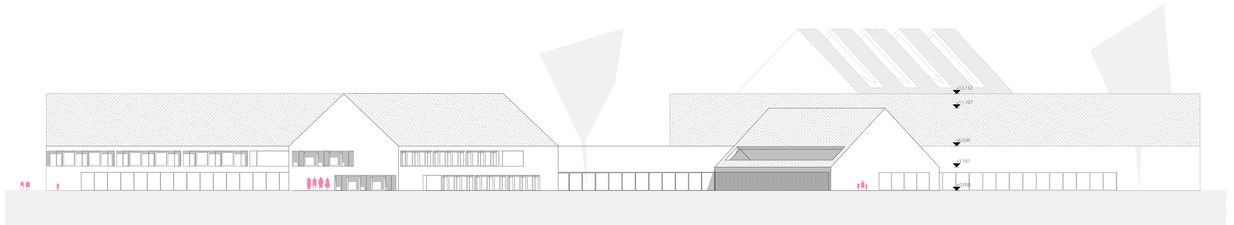
ÉSZAKNYUGATI HOMLOKZAT 1_250
