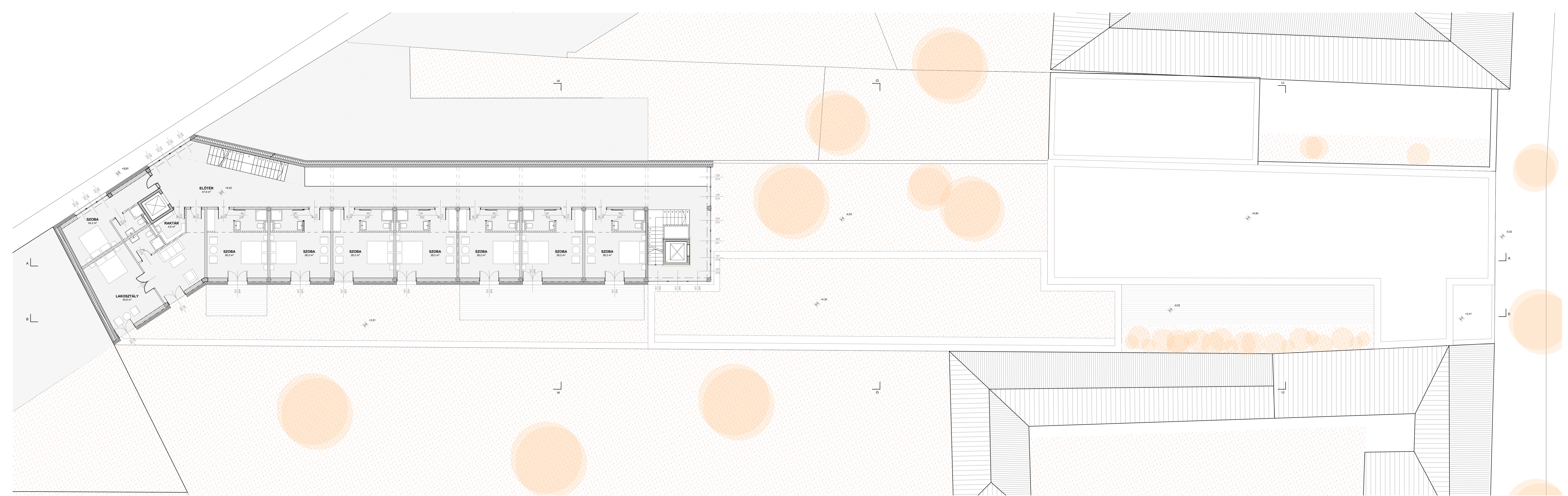
3. SZINT ALAPRAJZ M=1:100
