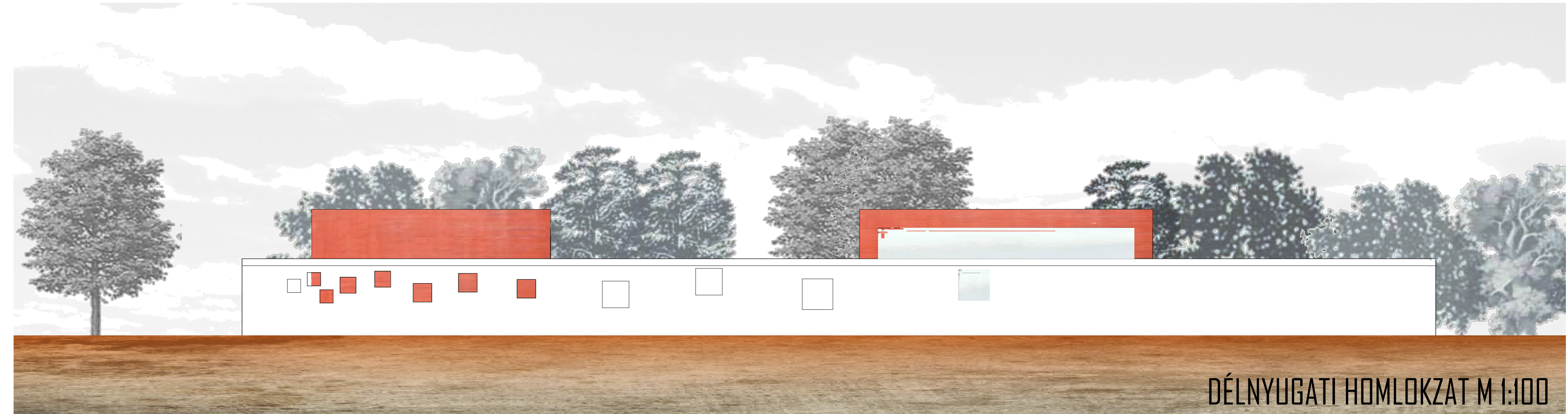
DÉLNYUGATI HOMLOKZAT - UDVARBAN M 1:100
