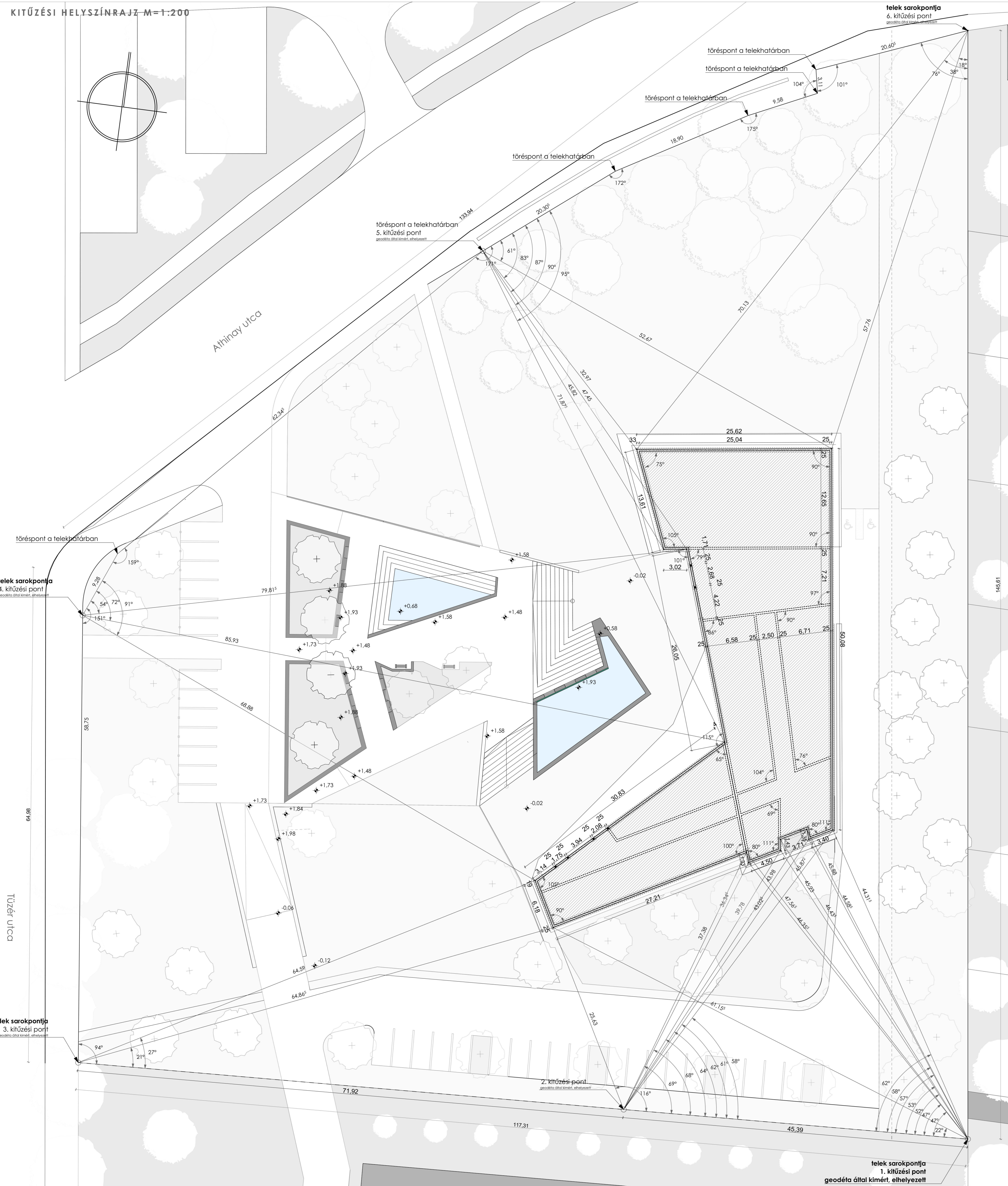
KITÜZÉSI HELYSZÍNRAJZ M=1:200
