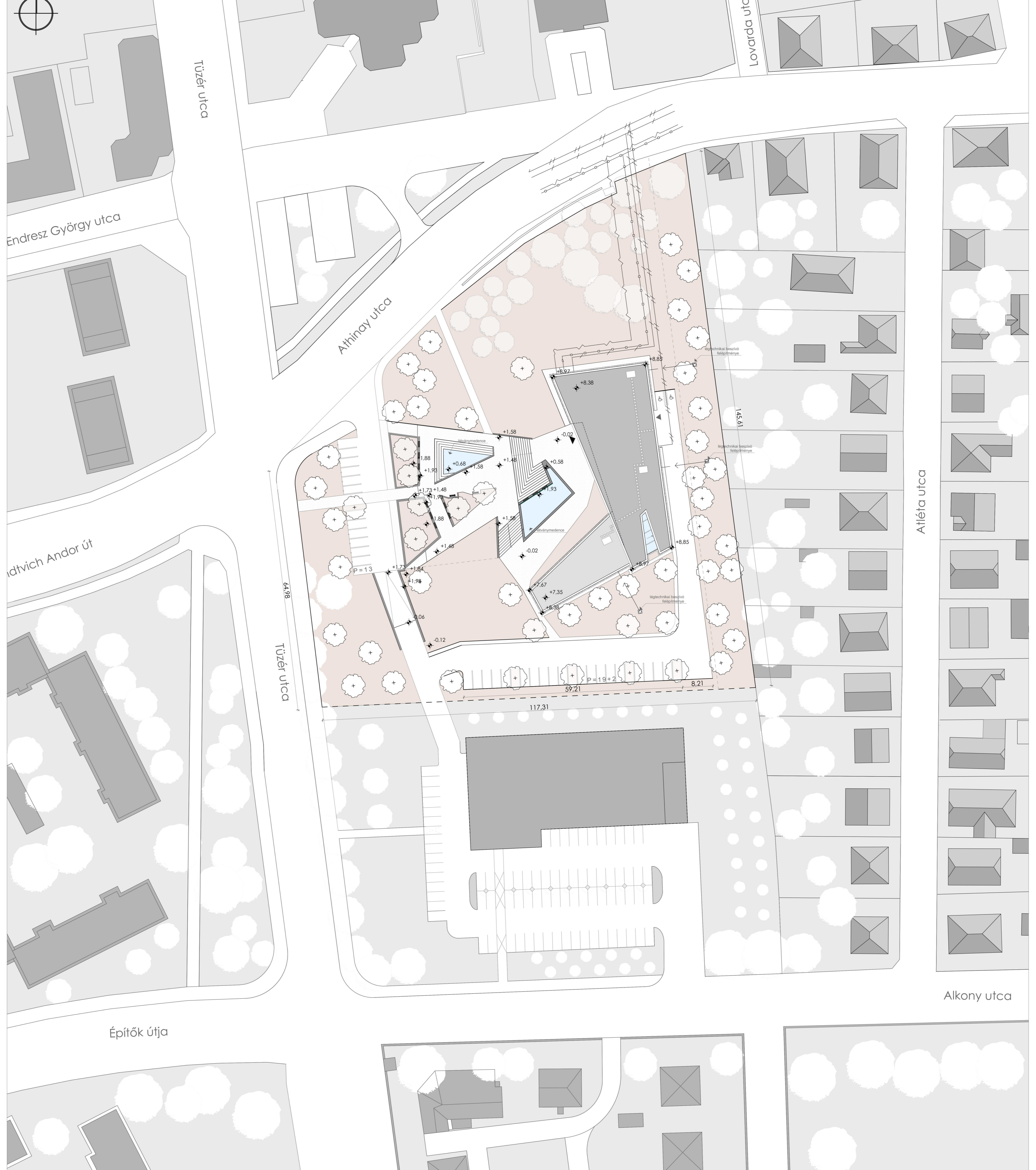
HELYSZÍNRAJZ M=1:500
