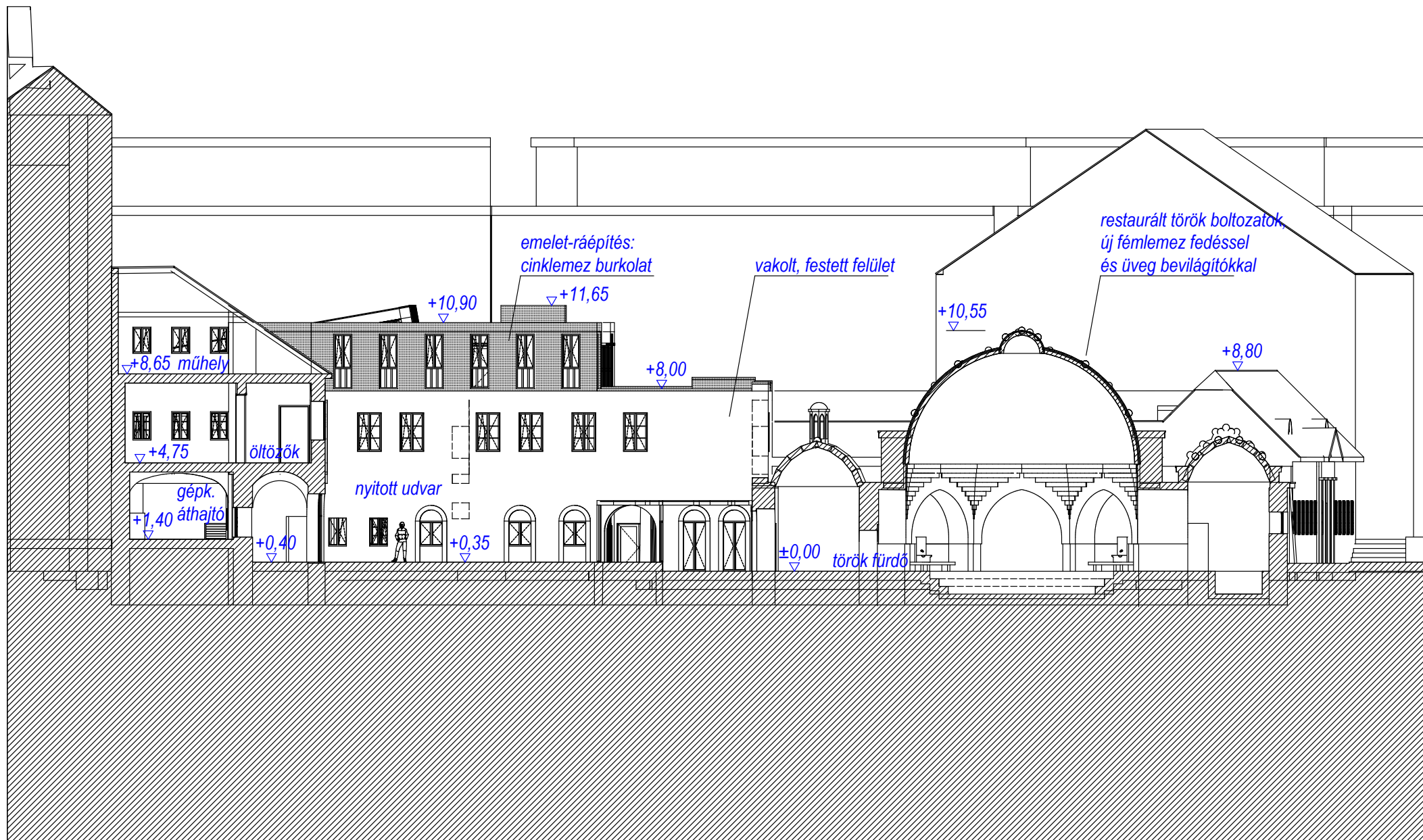
A-A METSZET M=1:200
