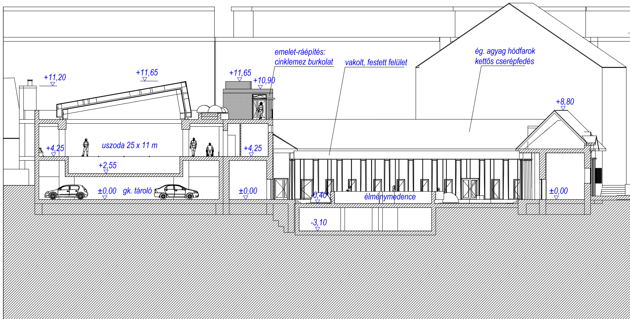
C-C METSZET M=1:200
