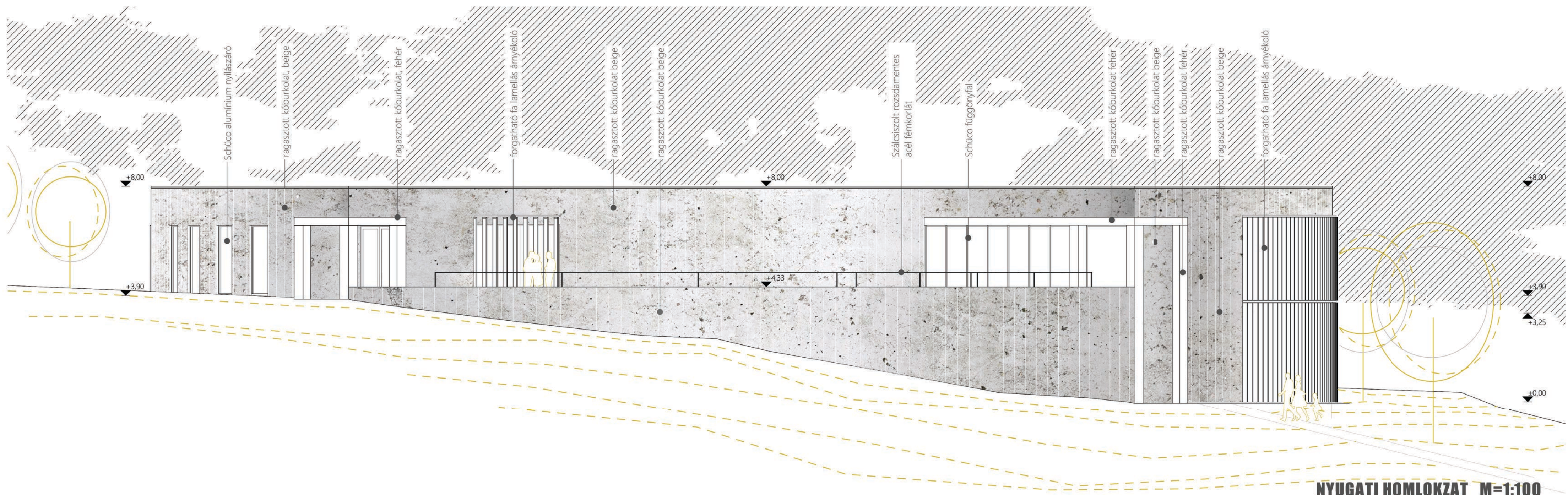
NYUGATI HOMLOKZAT_M=1:100
