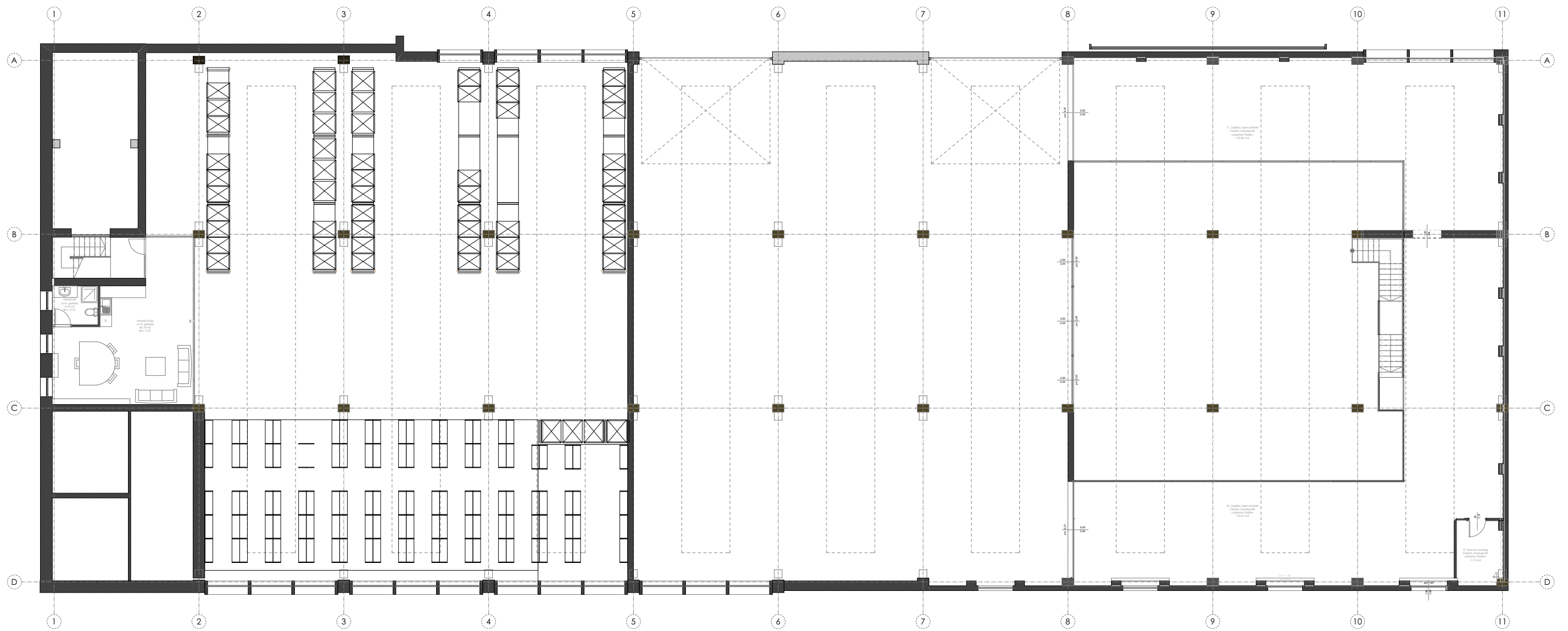
GALÉRIA ALAPRAJZ 1:100
