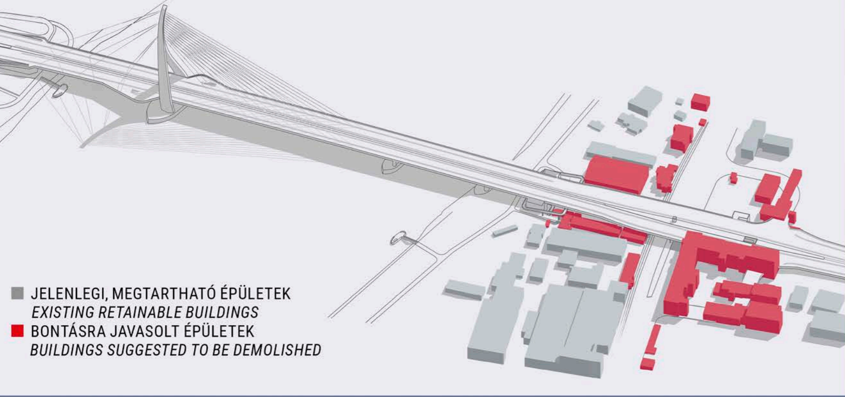
A TERVEZETT HÍD, A HOZZÁ KAPCSOLÓDÓ CSOMÓPONT, VALAMINT A BUDAFOKI ÚT SZÉLESÍTÉSE MIATT IGÉNYBEVETT TERÜLETEK / REQUIRED AREA OF THE PLANNED BRIDGE, RELATED TRAFFIC JUNCTION AND TO WIDEN BUDAFOKI ROAD
