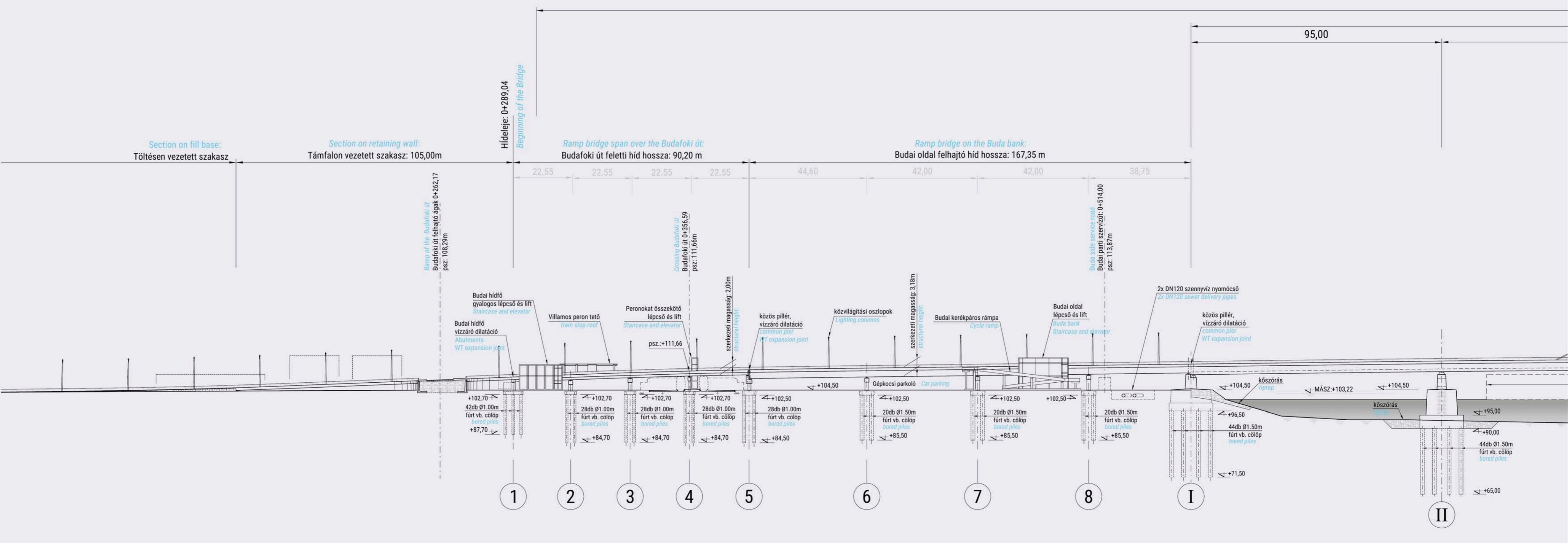
HOSSZMETSZET M 1:1000 / LONGITUDINAL SECTION SCALE 1/1000
