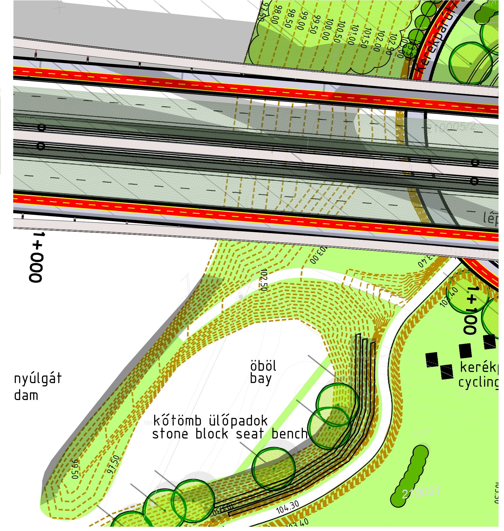
CSEPEL SIDE - CSEPELI OLDAL 1:500
