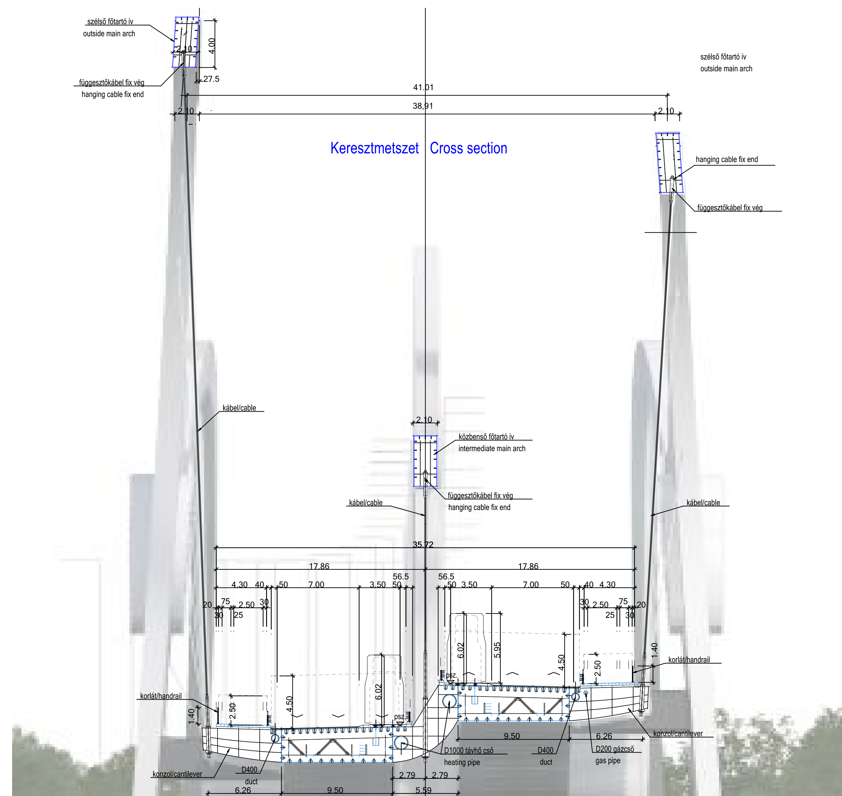
CROSS SECTION 'B' - KERESZTMETSZET "B" 1:200
