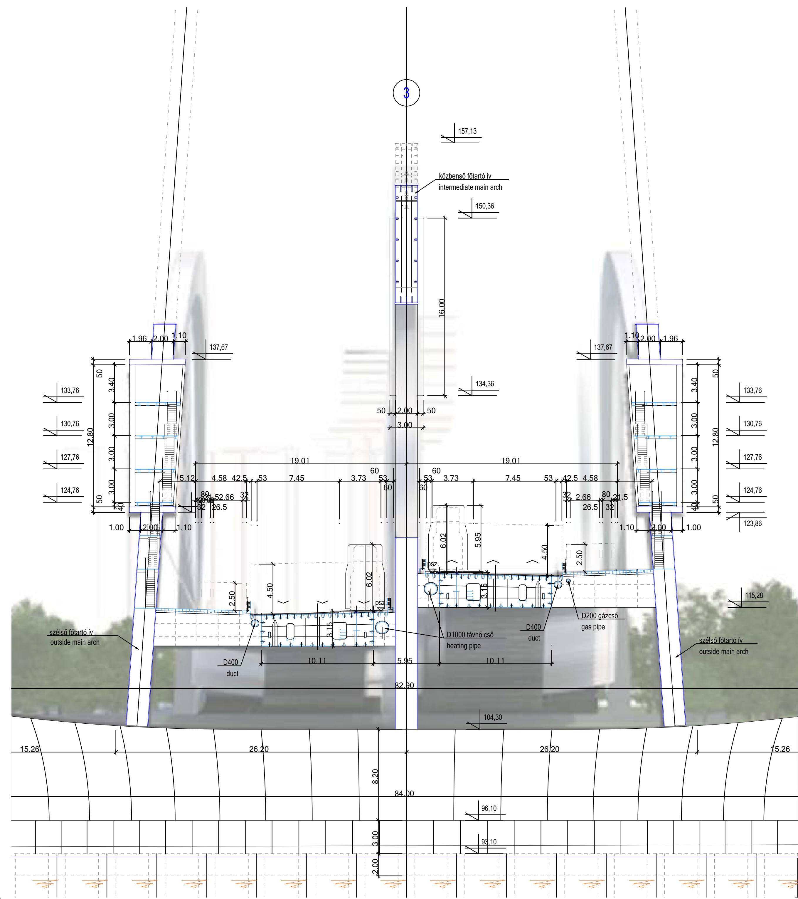
CROSS SECTION 'B' - KERESZTMETSZET "B" 1:200
