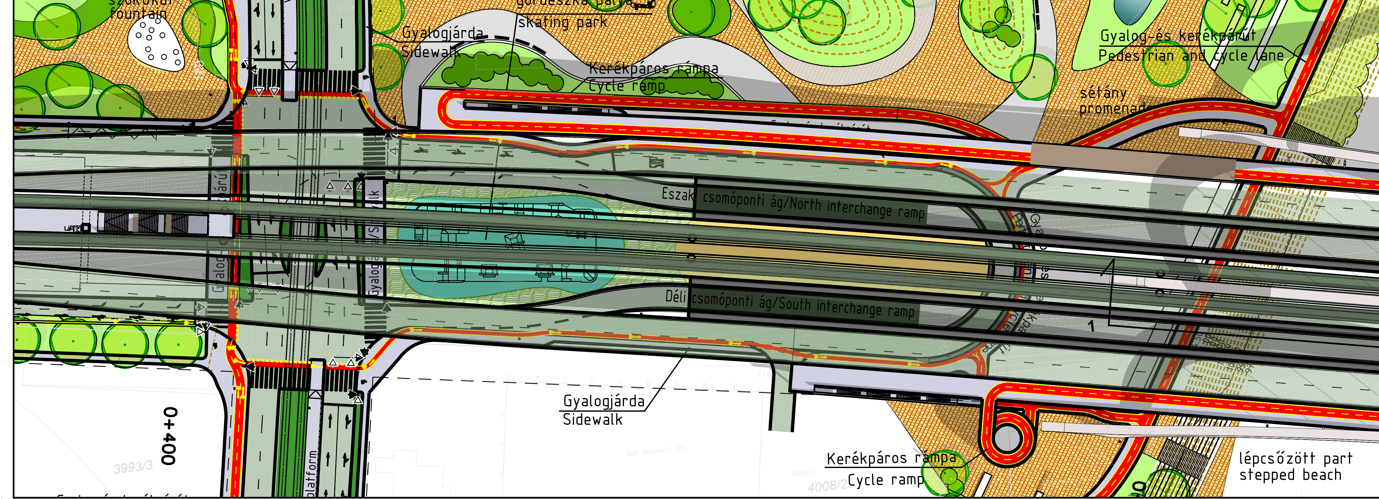
SITE PLAN DETAIL - ALAPRAJZI RÉSZLET 1:500
