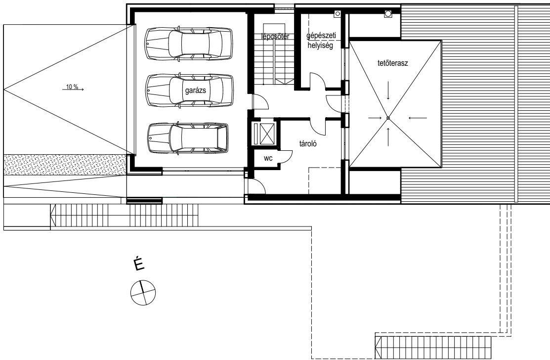
felső szint
