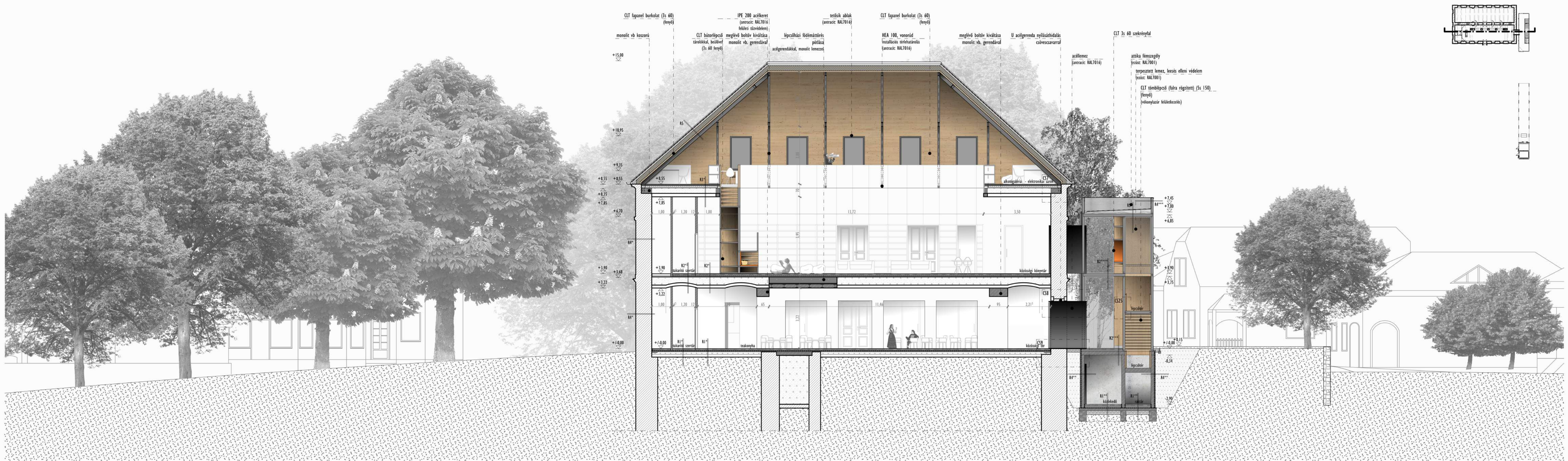
B - B metszet (kastély hosszmetset) M1:100
