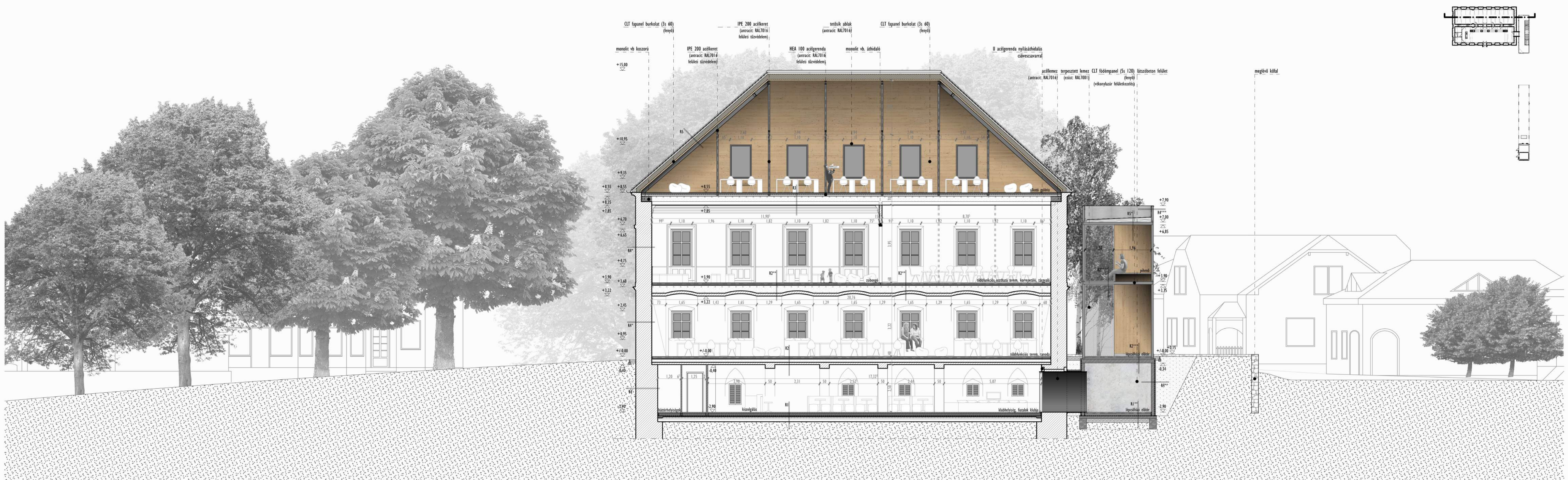
B - B metszet (kastély hosszmetset) M1:100
