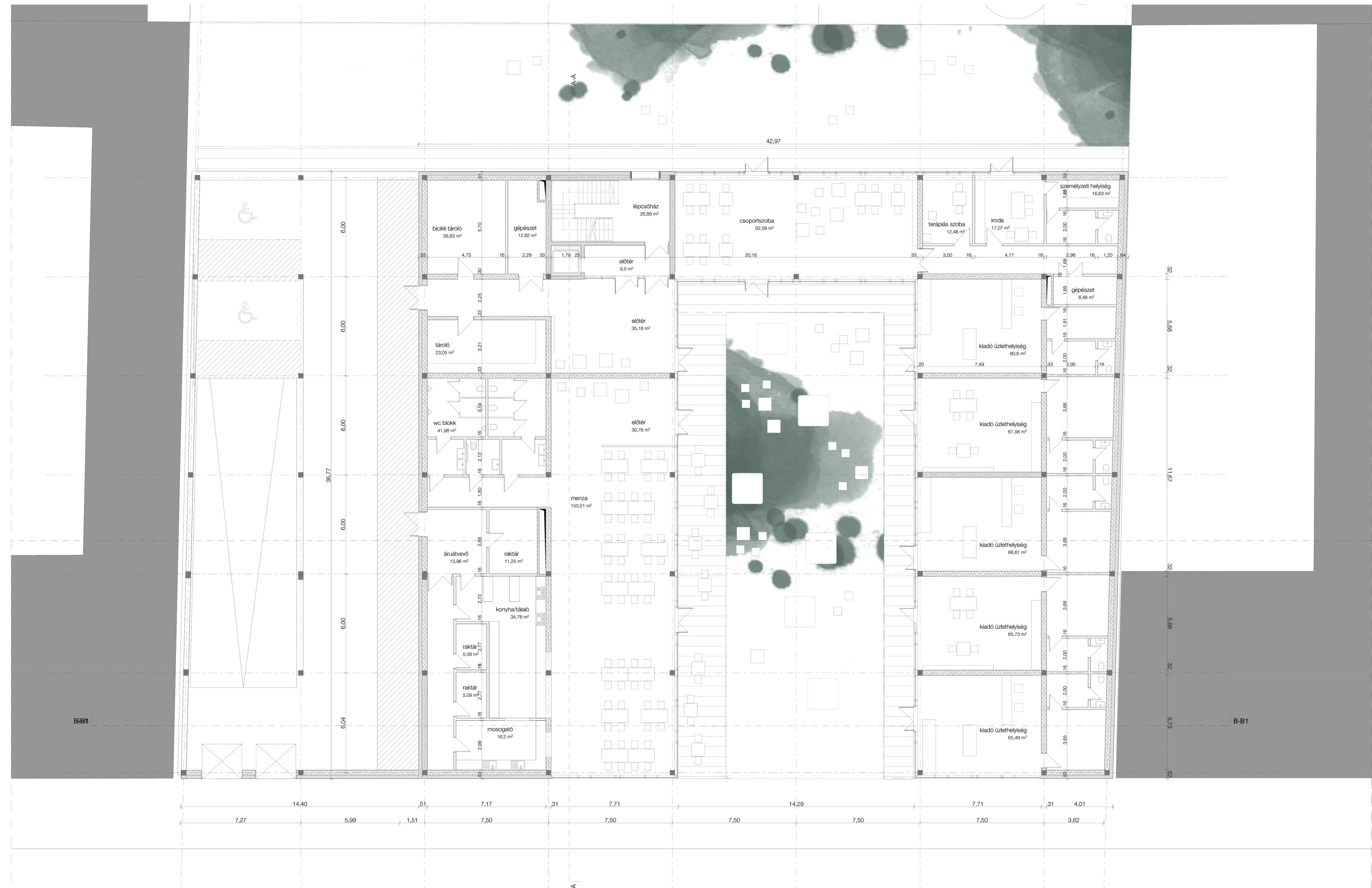
FÖLDSZINT ALAPRAJZ
