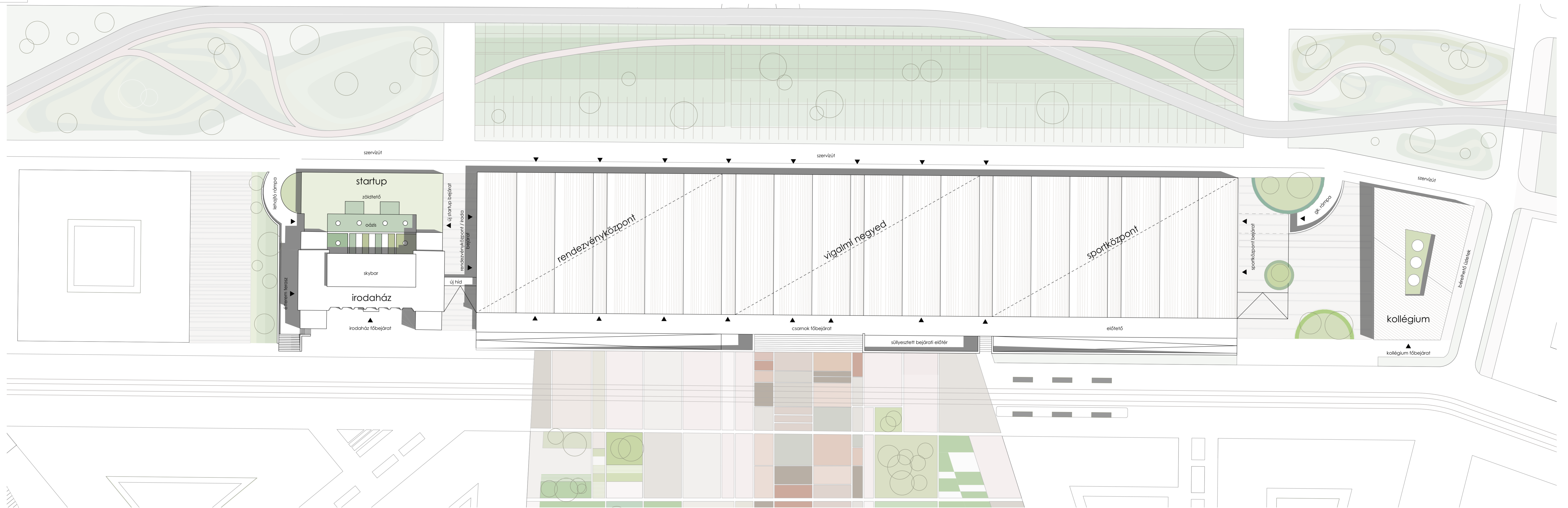
Helyszínrajz 1:500
