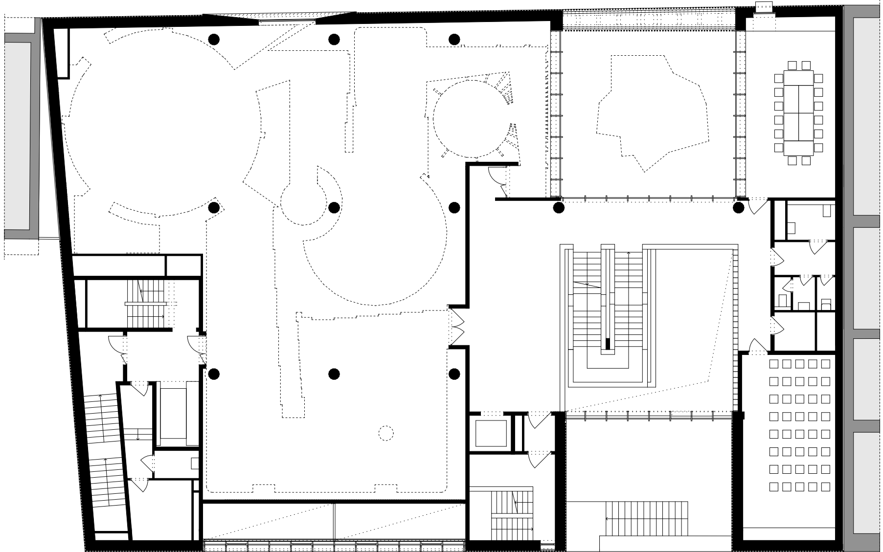
1. emeleti alaprajz
