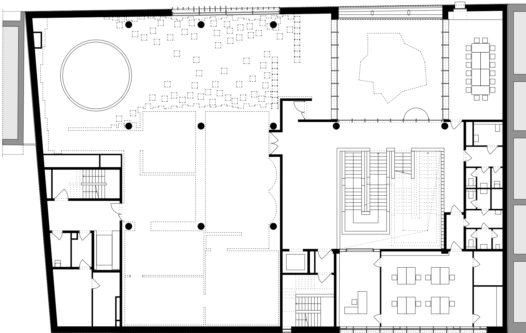
2. emeleti alaprajz
