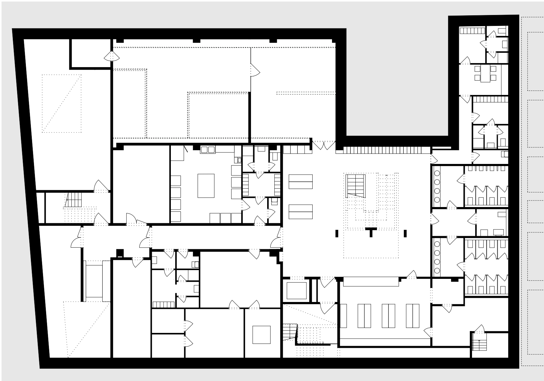
pinceszinti alaprajz
