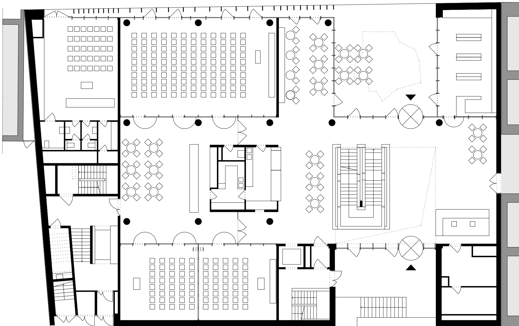
földszinti alaprajz
