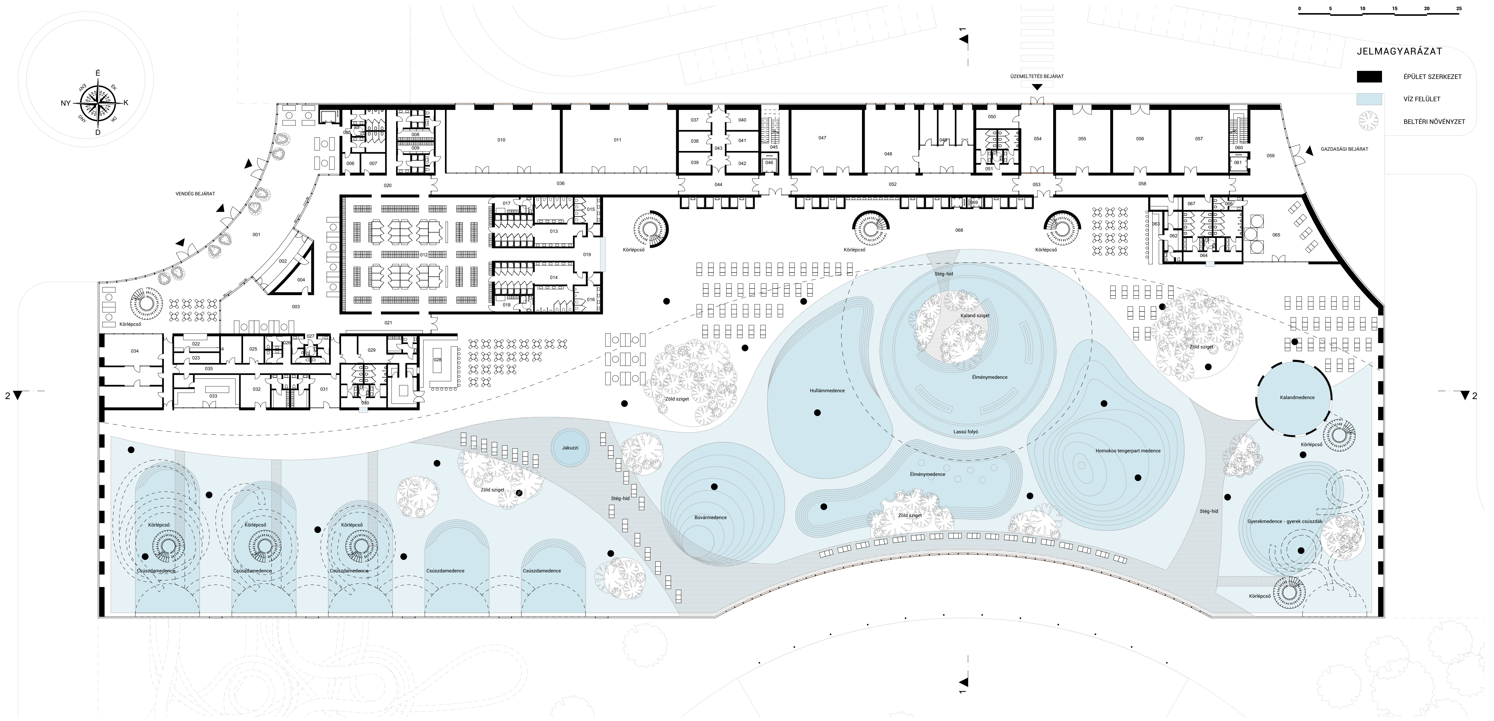
AQUAPARK - FÖLDSZINTI ALAPRAJZ M 1:350
