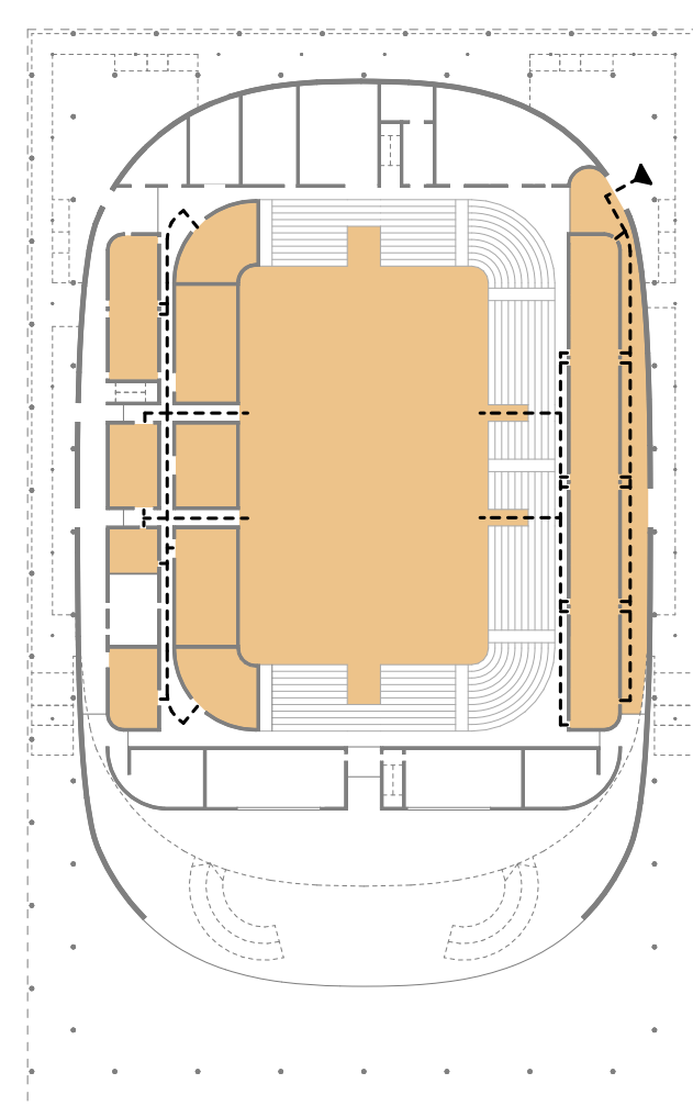
FÖLDSZINTI ALAPRAJZ
