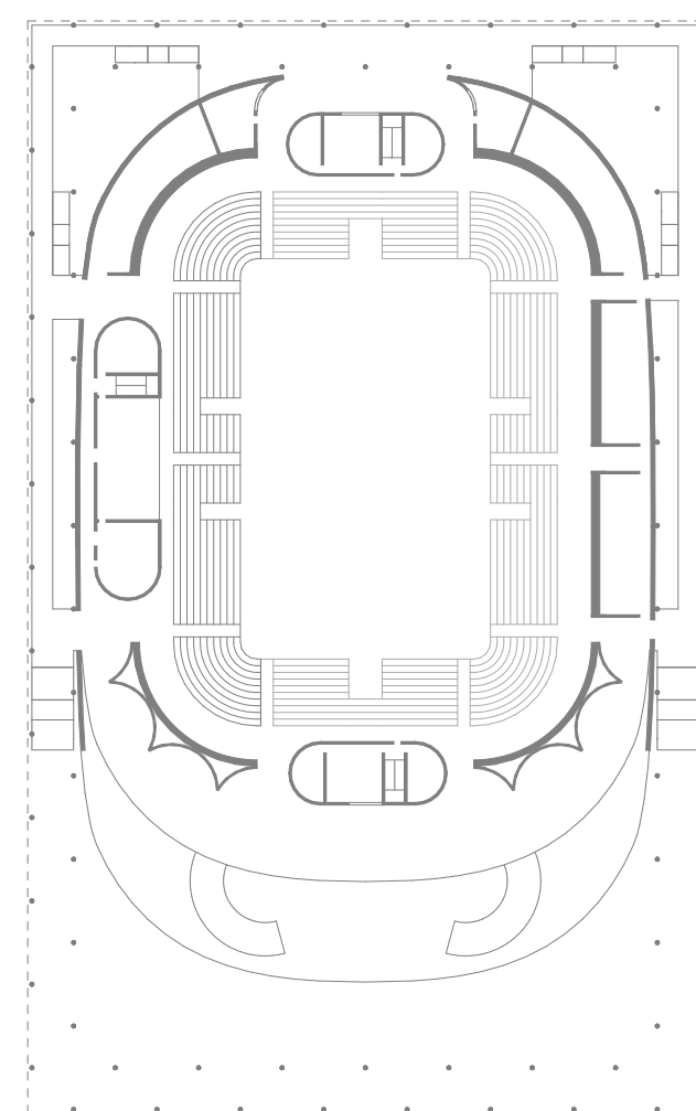
EMELETI ALAPRAJZ
